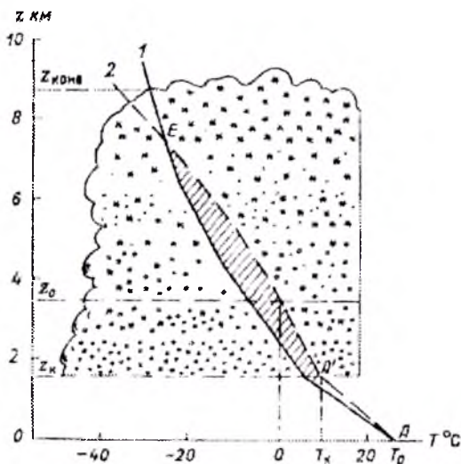
Рис. 28. Схема кучево-дождевого облака. 1 – кривая стратификации, 2 – кривая состояния.
