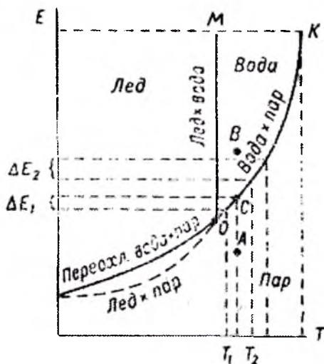
Рис. 25. Зависимость давления насыщения от температуры и фазового состояния испаряющей поверхности.
