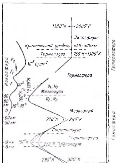
Рис. 1. Схема вертикального строения атмосферы
