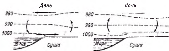
Рис. 42. Схема бризов.
