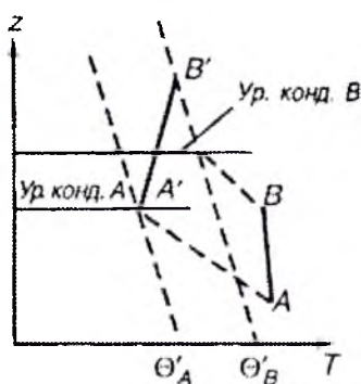
Рис. 12. Потенциальная устойчивость
