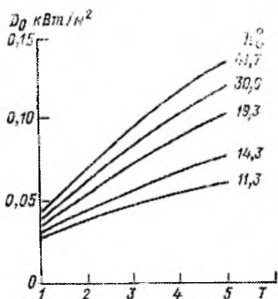
Рис. 16. Зависимость интенсивности рассеянной радиации при безоблачном небе от фактора мутности T при различной высоте солнца h_{\odot} .
