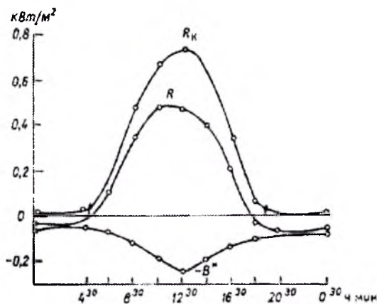
Рис. 17. Суточный ход радиационного баланса R и его коротковолновой R_k и длинноволновой составляющих (Юг Казахстана, июль 1952 г.).
