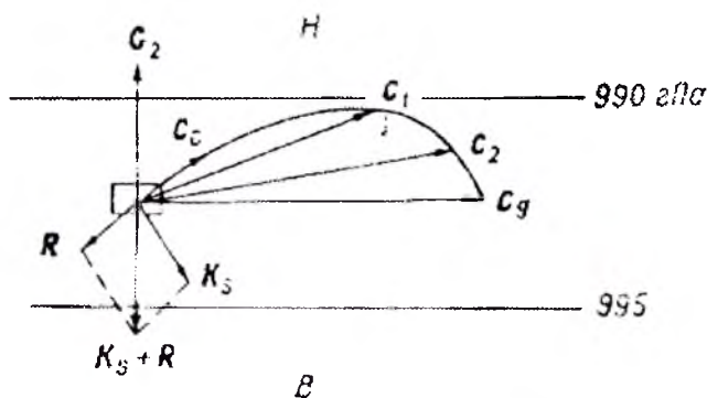
Рис. 40. Распределение скорости и направления ветра с высотой в пограничном слое атмосферы (северное полушарие).
