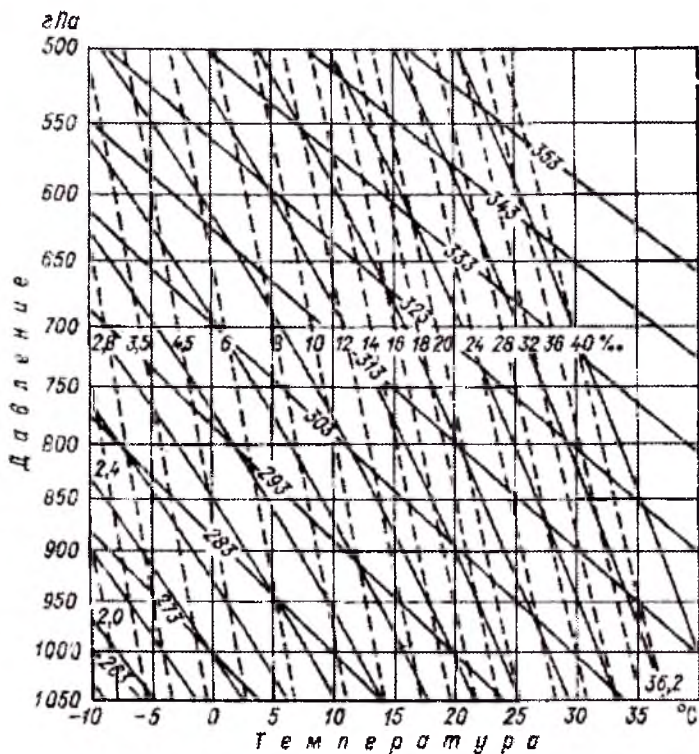
Рис. 13. Аэрологическая диаграмма.
