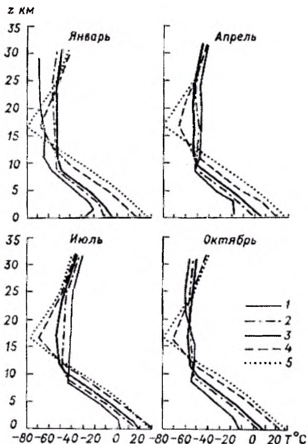
Рис. 23. Распределение средней (за месяц) зональной температуры с высотой.
