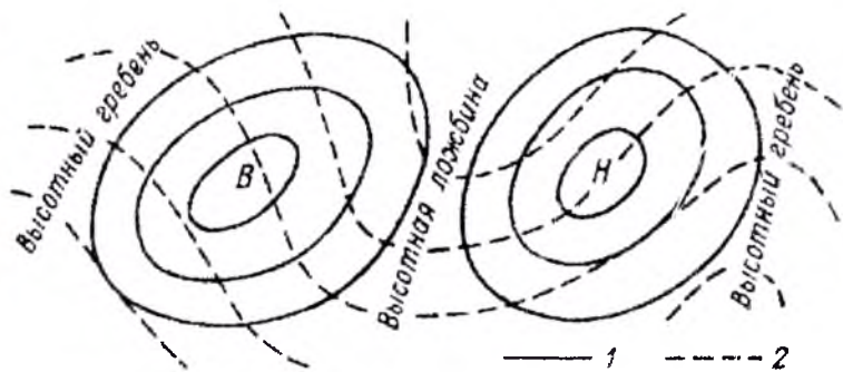
Рис. 5. Изобары в циклоне (H) и антициклоне (B) на уровне моря (1) и в высоких слоях (2).
