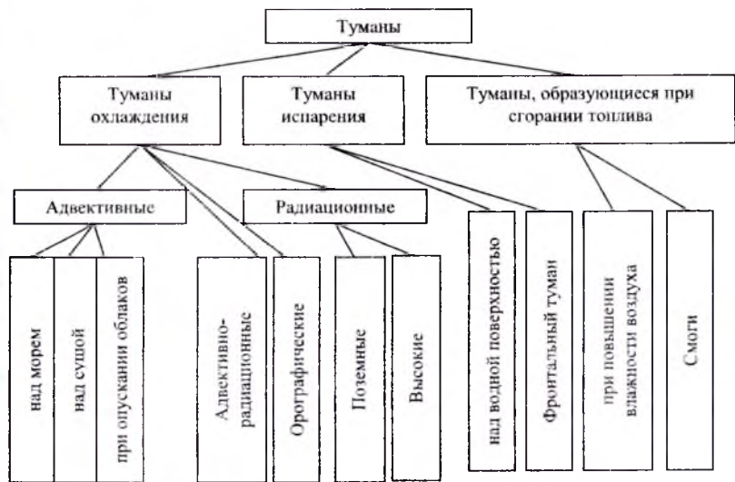
Рис. 27. Схема классификации туманов.
