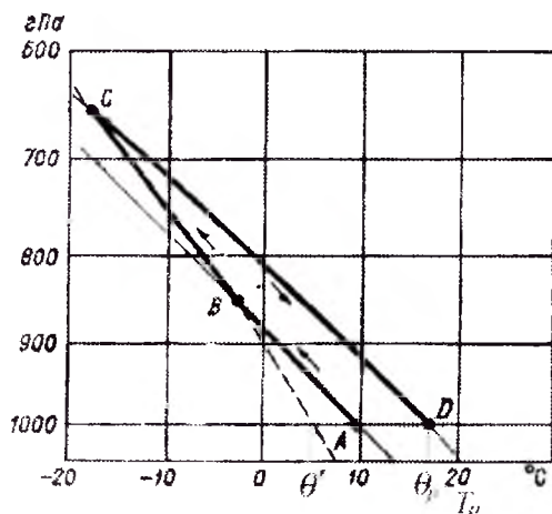
Рис. 9. Псевдоадиабатический процесс.
