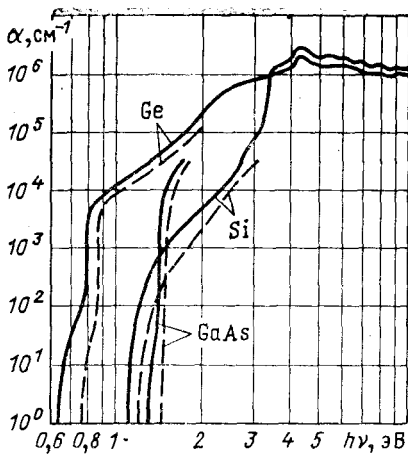
Рис. 11.8. Спектр поглощения чистых Ge, Si, GaAs
