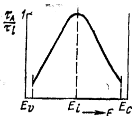
Рис. 7.5. Время жизни при ударной межзонной рекомбинации в зависимости от положения уровня Ферми
