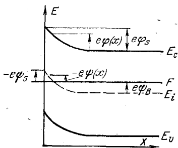
Рис. 10.4. Энергетическая диаграмма поверхностной области полупроводника n -типа
