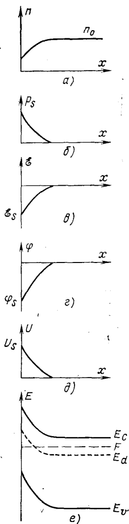
Рис. 9.3. Концентрация свободных электронов (а), плотность объемного заряда (б), напряженность электрического поля (в), потенциал поля (г), потенциальная энергия электронов (д) и искривление зон донорного полупроводника (е) при изменении направления внешнего электрического поля
