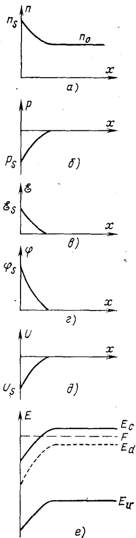
Рис. 9.2. Изменение концентрации свободных электронов (а), объемного заряда (б), напряженности поля (в), потенциала поля (г), потенциальной энергии электронов (д) и искривление зон донорного полупроводника (е) во внешнем электрическом поле
