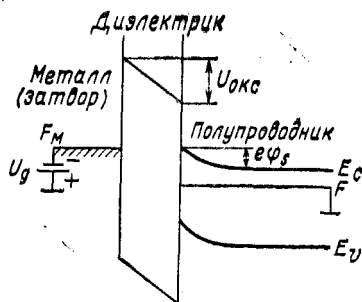
Рис. 10.9. Энергетическая диаграмма структуры, изображенной на рис. 10.8
