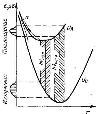
Рис. 12.1. Схема энергетических уровней примесного центра в твердом теле
