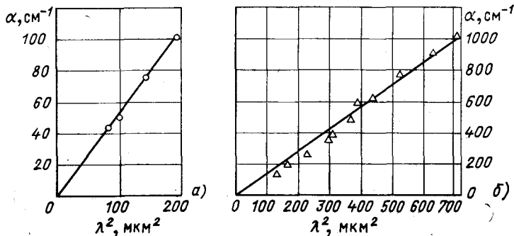
Рис. 11.28. Зависимость коэффициента поглощения InSb n -типа от квадрата длины волны для концентрации электронов 3,5 \cdot 10^{17} (а) и 6,2 \cdot 10^{17} \text{ см}^{-3} (б)
