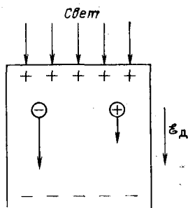
Рис. 13.11. Возникновение ЭДС Дембера
