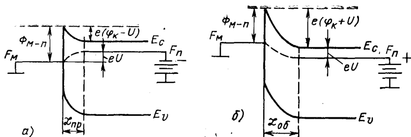
Рис. 9.8. Контакт металл-дырочный полупроводник в случае \Phi_M > \Phi_{II} (a) и \Phi_M < \Phi_{II} (б)
