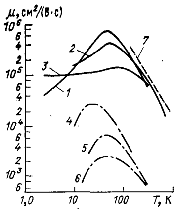
Рис. 6.2. Температурные зависимости подвижности электронов и дырок в антимиониде индия: 1 — n = 2 \cdot 10^{14} ; 2 — n = 10^{15} ; 3 — n = 10^{16} \text{ см}^{-3} ; 4 — p = 3 \cdot 10^{14} ; 5 — p = 4 \cdot 10^{15} ; 6 — p = 3 \times 10^{16} \text{ см}^{-3} ; 7 — теоретические значения подвижности электронов
