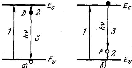
Рис. 12.11. Излучательные переходы между зоной и примесными состояниями
