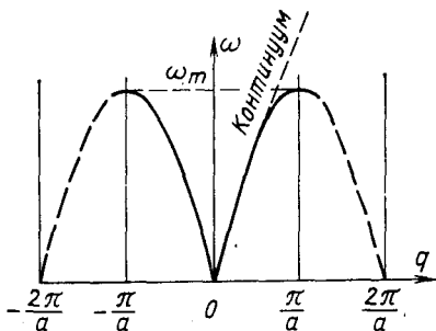
Рис. 3.2. Зависимость частоты колебания от волнового числа для линейной решетки, состоящей из одинаковых атомов, и для упругой струны
