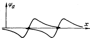
Рис. 2.9. Атомные функции p -состояния, описываемые уравнением (2.81)
