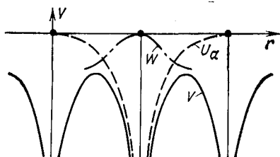
Рис. 2.1. Схематическое изображение периодического потенциала одномерной решетки. Сплошная кривая — потенциал решетки V(\mathbf{r}) ; пунктирная — атомный потенциал U_a(\mathbf{r}) ; штрихпунктирная — возмущающий потенциал W(\mathbf{r})
