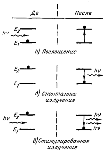
Рис. 12.16. Три основных типа переходов между энергетическими уровнями E_1 и E_2 :
