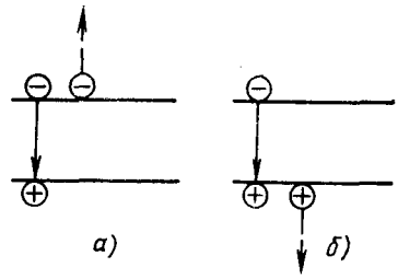
Рис. 7.4. Схема процессов межзональной ударной рекомбинации
