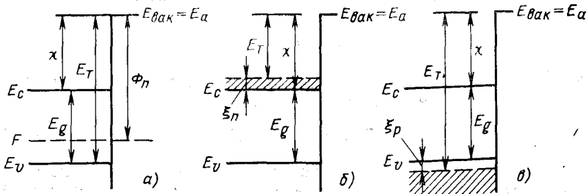
Рис. 13.20. Зависимость внешнего фотоэффекта от степени легирования полупроводника
