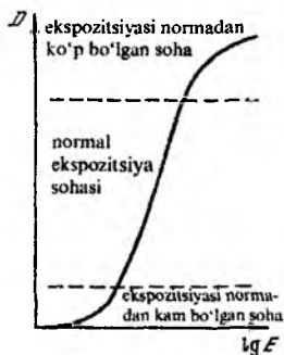
69-rasm. Fotomaterialning xarakteristik egriligi
