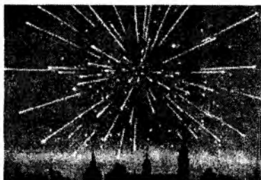
117-rasm. «Uchar yulduz»lar va ularning radianti
