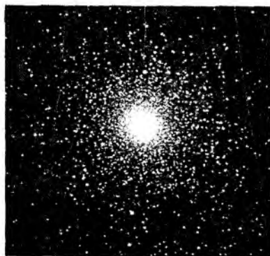
151-rasm. Gerkules yulduz turkumidagi sharsimon yulduz to'dasi
