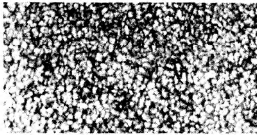
79-rasm. Quyosh fotosferasining donodorlik strukturasi
