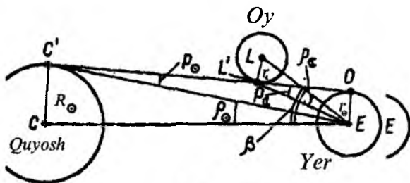
48-rasm. Quyoshning tutilish shartlarini tushuntiruvchi chizma
