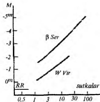
141-rasm. Sefeidlar va Liraning RR tipidagi yulduzlar yorqinliklari
