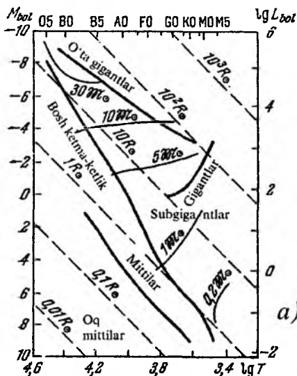
127-rasm. Radius – yorqinlik-massa diagrammasi (a) va massasi hamda radiuslari ularga mos yulduzlar (b)
