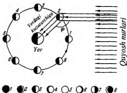
44-rasm. Oy fazalarining Quyoshga va Yerga nisbatan turli holatlari
