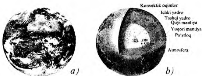
95-rasm. Yerning sirtqi va ichki tuzilishi
