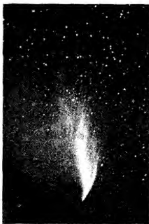
115-rasm. «Dumli yulduz»ning yulduzlar fonida ko'rinishi
