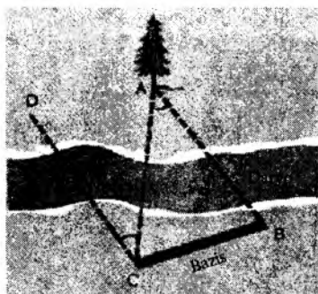
34-rasm. Yer sirtida borib bo'lmaydigan obyektga qadar masofani hisoblash usuli
