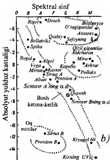
127-rasm. Radius – yorqinlik-massa diagrammasi (a) va massasi hamda radiuslari ularga mos yulduzlar (b)
