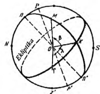
6-rasm. Ekliptikal koordinatalar sistemasi
