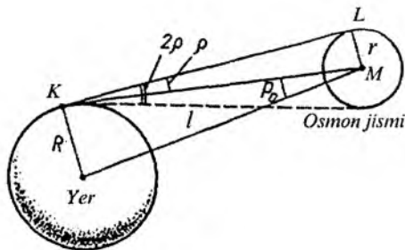
37-rasm. Quyosh sistemasi jismlarining chiziqli o'lchamlarini hisoblash.
