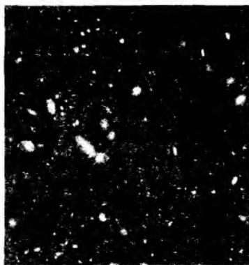
159-rasm. Osmonning 1 kv. gradus maydoniga to'g'ri keladigan galaktikalari
