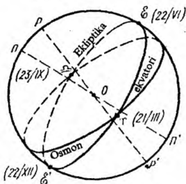
3-rasm. Ekliptikaning osmon ekvatoriga nisbatan joylashishi
