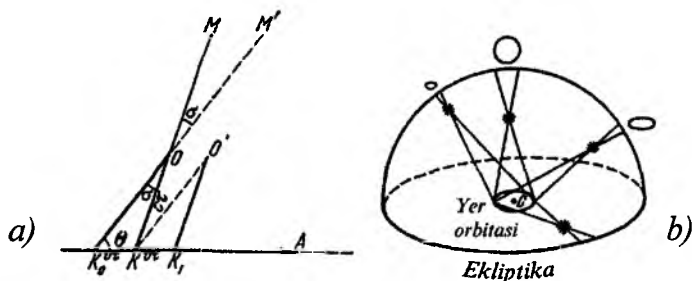
39-rasm. Yoritgichlarning yillik parallaksini aniqlash
