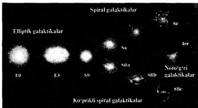
157-rasm. Galaktikalar evolyutsiyasining kechishi
