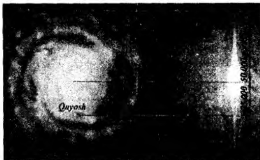
147-rasm. Galaktikamiz va unda Quyoshning o'rni
