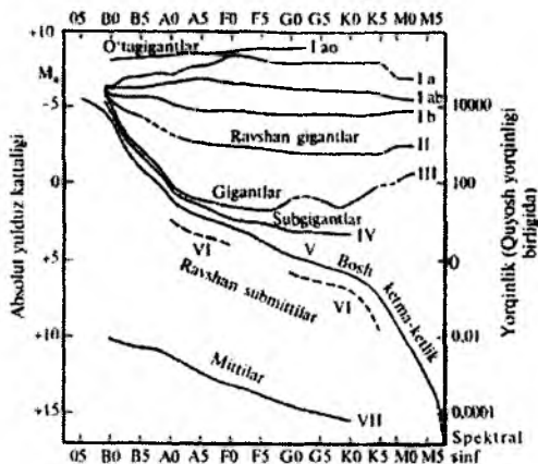
124-rasm. Yulduzlarning yorqinliklari bo'yicha sinflarga bo'linishi
