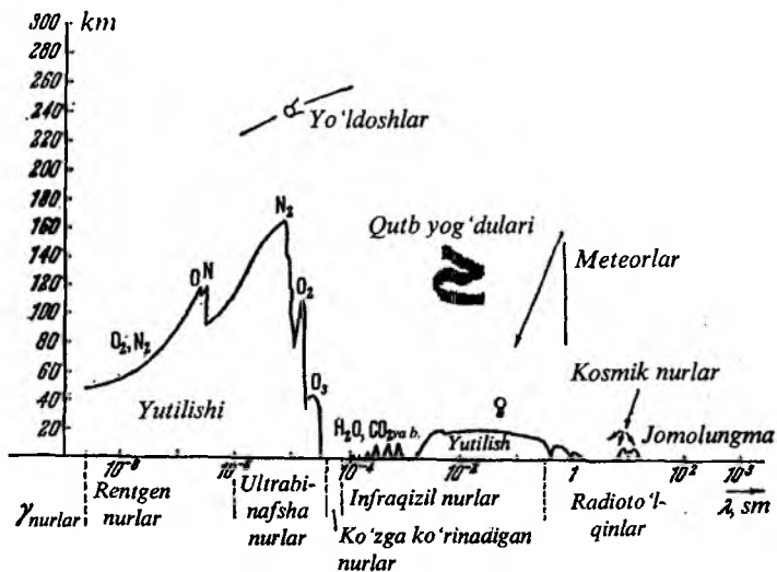
52-rasm. Yer atmosferasida turli to'liq uzunligidagi nurlarning yutilishi
