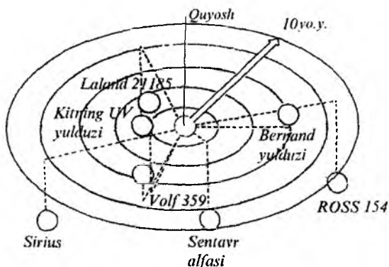
121-rasm. Quyoshdan 10 yorug'lik yilgacha masofada bo'lgan yulduzlar
