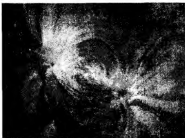
88-rasm. Xromosfera chaqnashlari
