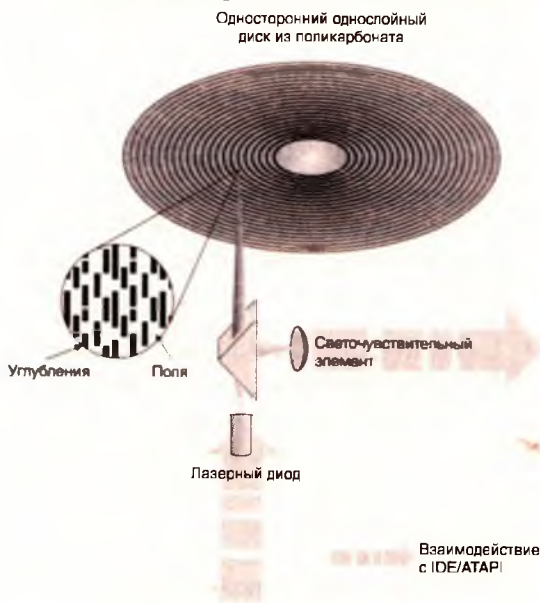
Рис. 3.4. Принцип действия дисковода CD-ROM
