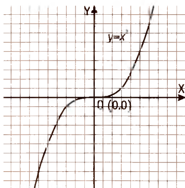
Рис. 15.5. Кривая третьего порядка (слева) и кривая Безье (справа)
