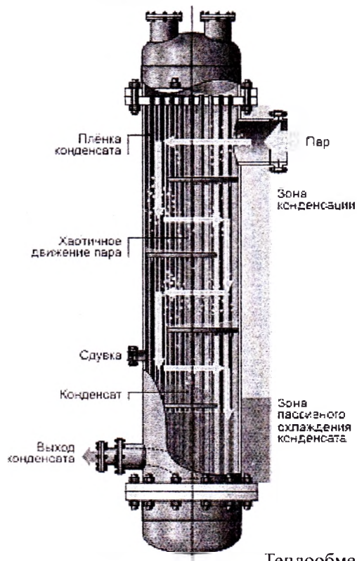
Стандартный теплообменник
