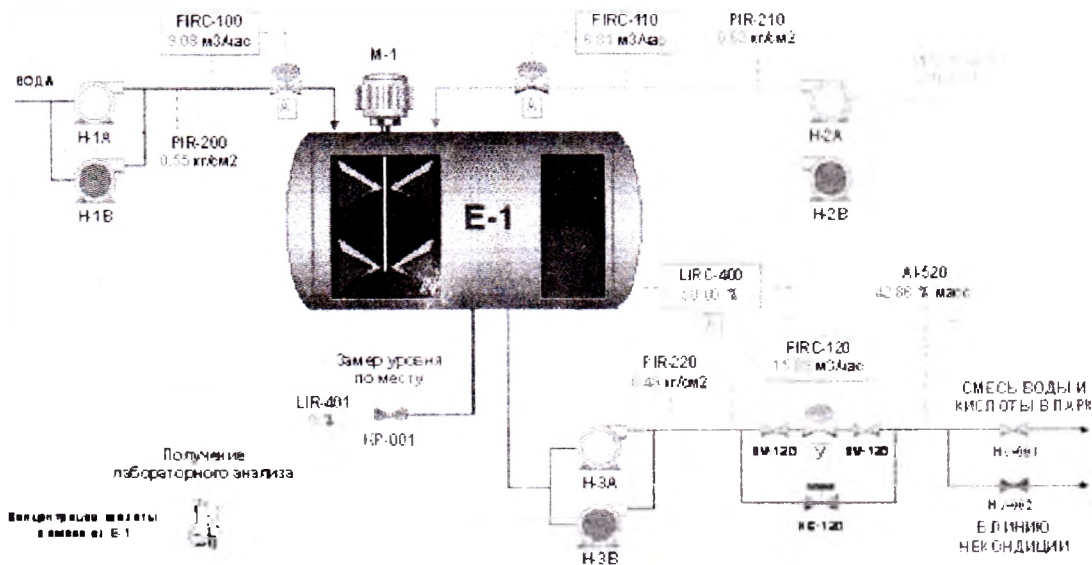
Рис. 6.1. Схема узла смешения.
