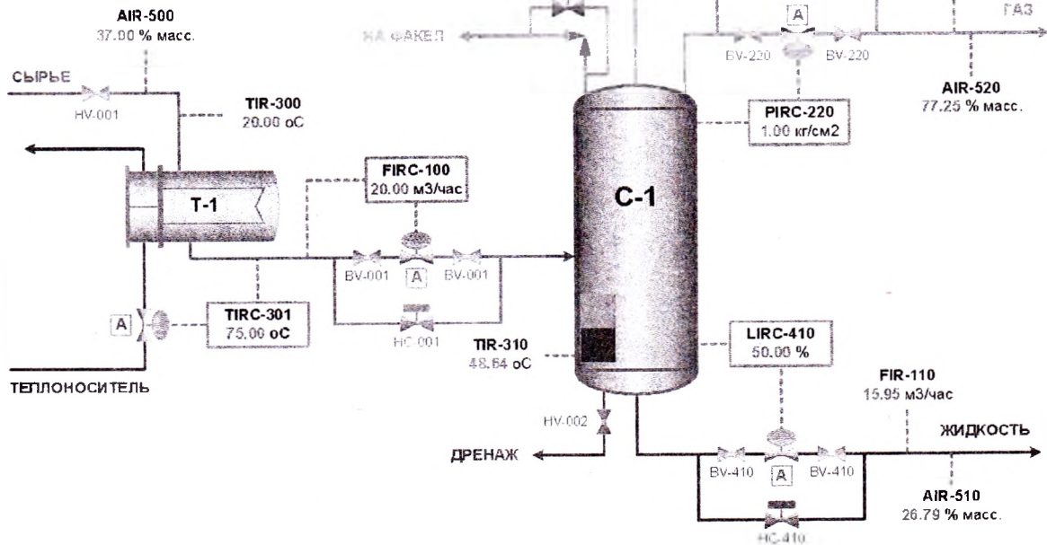
Рис. 8.1. Схема узла сепарирования
