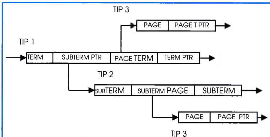
7.18-расм. Предмет кўрсаткичини тақдим этадиган кўп боғли рўйхат ёзувларишнинг форматлари
