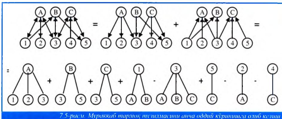
7.5-расм. Мураккаб тармоқ тузилмасини анча oddий кўринишга олиб келиши
