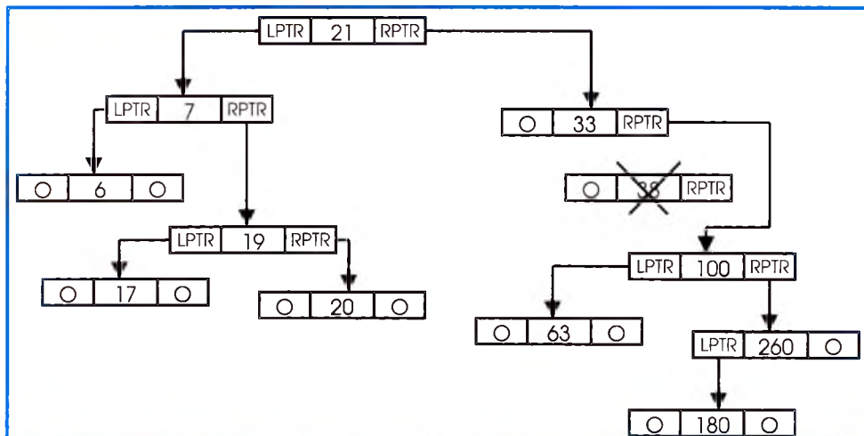
7.15-расм. Икки боғли рўйхатга элементларни киритиши ва undan чиқариб ташлаши
