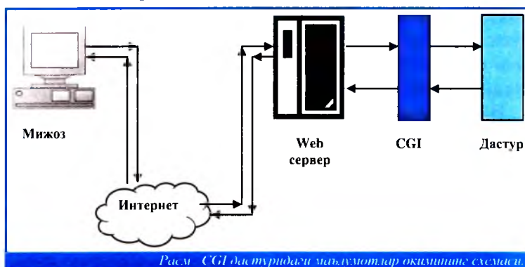
Рис. CGI дастуридаги маълумотлар оқинише схемаси
