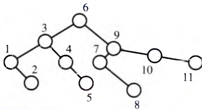
10.7-расм. Саралаштириш мувозанатлаштирилган иккиланган дарахти
