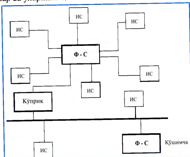
3.9-расм. Тармоқларнинг жисмоний имкониятларини кенгайтириши
