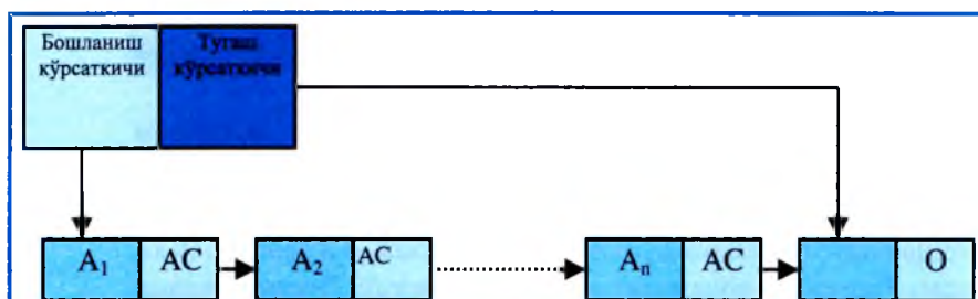
6.6-расм. Навбатни боғланган таъдим этиши
