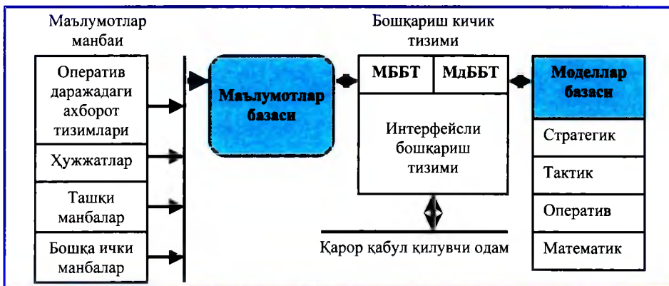
2.17 расм. Қарорлар қабул қилишни қўллаб-қувватлаш ахборот технологияларининг асосий компонентлари
