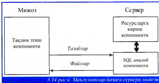
3.14-расм. Маълумотлар базаси сервери модели
