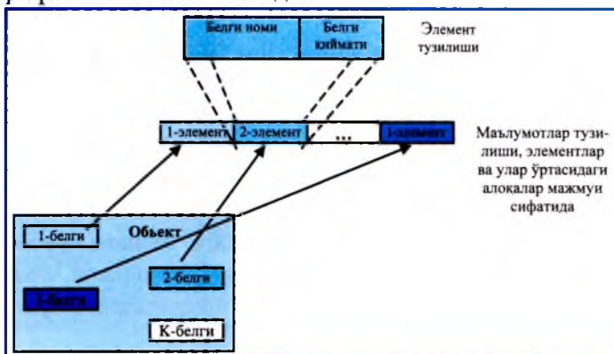
5.1 расм. Объект ва маълумотлар тузилмаси ўртасидаги ўзаро боғлиқлик
