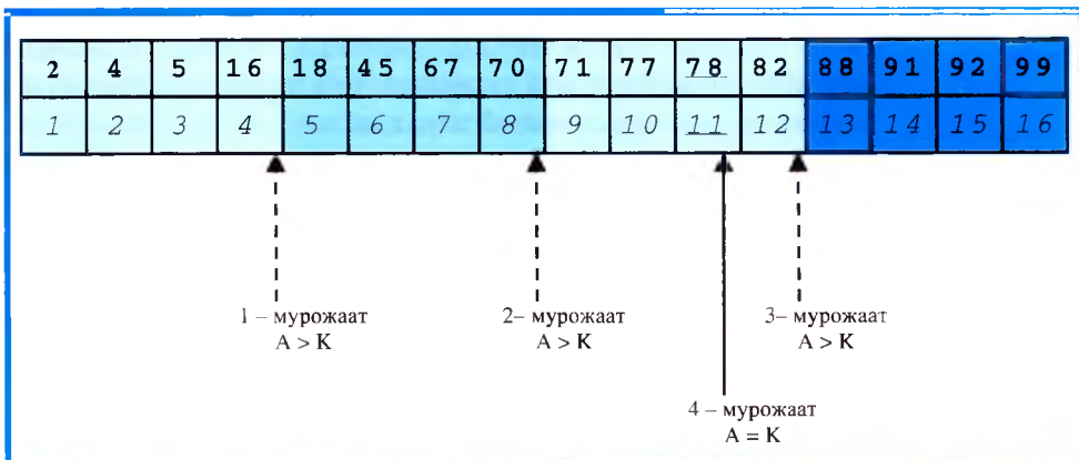
11.2-расм. Блокли излаш схемаси
