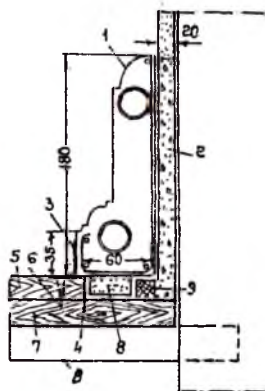
4.12-rasm. Plintusga o'rnatilgan betondan quyilgan isitish asbobi: 1 – isituvchi panel; 2 – issiqlik saqlovchi material; 4 – karton; 5 – parket; 6 – burma mix; 7 – qora pol; 8 – qum qatlami; 9 – yog'och to'sini.
