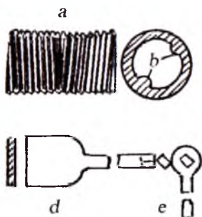
4.2-rasm. Nippel va radiator seksiyalarini birlashtirish uchun qo‘llaniladigan kalit: a – nippel; b – nippelni burab yurguzuvchi ko‘ndalang valik; d – radiator uchun kalit; e – yoqalik kalit
