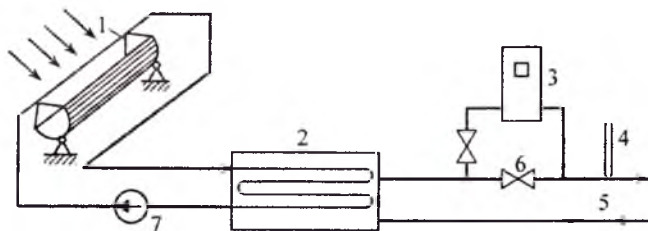
15.8-rasm. Parabolosilindrik konsentratli va suyuq issiqlik yig'uvchi moslamali past haroratli isitish tizimi: 1 – parabolosilindrik konsentrat; 2 – suyuqlikli issiqlik akkumulyator; 3 – qo'shimcha issiqlik manba; 4 – termometr; 5 – isitish tizimi konturi; 6 – boshqaruvchi jo'mrak; 7 – uyurmaviy nasos
