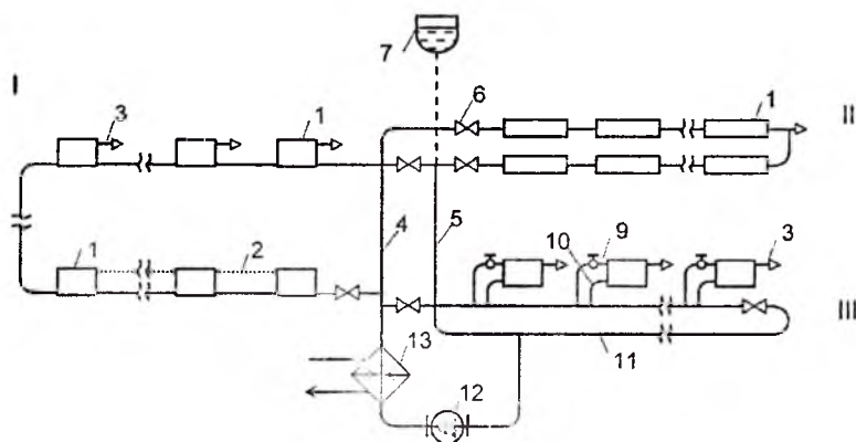
7.5-rasm. Bir quvurli gorizonttal (ko'ndalang) isitish tizimidagi isitish asboblarni taqsimlovchi magistral quvurlarga turli xil ulash sxemalari: I - gorizonttal (ko'ndalang) quyidan yuqoriga harakat qiluvchi isitish tizimi; II - quyidan yuqoriga harakat qiluvchi bifilyar isitish tizimi; III - oxirida birlashtiruvchi quvur bo'limi. 1 - isitish asbobi; 2 - havo quvuri; 3 - havo jo'mragi; 4 - taqsimlovchi tirgak; 5 - qaytuvchi tirgak; 6 - jo'mrak; 7 - kengaytiruvchi idish; 8 - konvektorlar; 9 - jo'mrak; 10 - tirgak; 11 - teskari magistral quvur; 12 - nasos; 13 - issiqlik almashgich (qozon)
