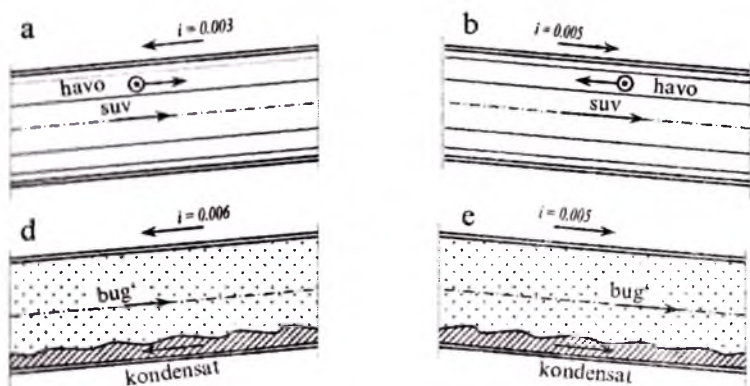
5.6-rasm. Isitish asbolarida issiqlik tashuvchining harakat yo'nalishi hamda taklif qilingan va ruxsat etilgan qiyalik darajasi: a va b – yuqoridan tarqatiluvchi issiq suvli isitish qurilmalarida; d va e – issiqlik tashuvchi bug' bo'lgan holda
