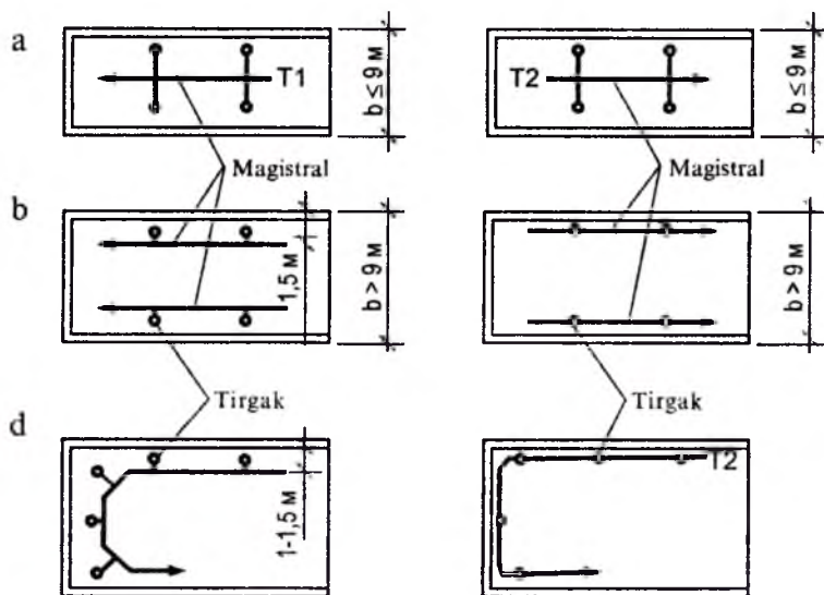
5.5-rasm. Magistral quvurlarining yerto'la va texnik qavatlarida o'rnatilishi: a – chordoqli binolarda; b – yerto'la va texnik qavatlarida; d – issiqlik tashuvchining yo'lma-yo'l harakat sxemasi
