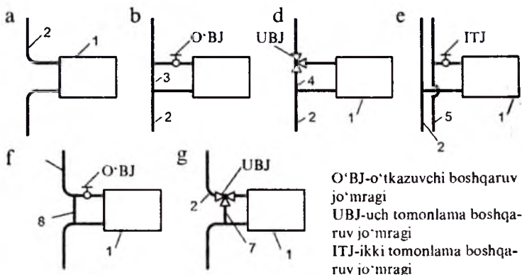
5.7-rasm. Bir (a-d) va ikki (e) quvurli vertikal isitish tizimida quvurlarning isitish asboblariга bir tomonlama ulanishi: 1 - isitish asboblari; 2 - bir quvurli tirgaklar, 3 - o'qi siljiltilmagan birlashtiruvchi tirgaklar; 4 - o'qli aylanma uchastkasi; 5 va 6 - ikki quvurli tirgaklarda isitish tizimlariga issiqlik uzatuvchi va qaytaruvchi quvurlar; 7 - o'qdan siljiltilgan tutashtiruvchi quvur; 8 - siljiltilmagan tutashtiruvchi quvur
