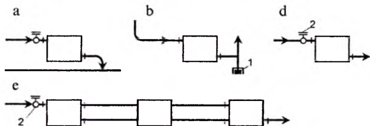
5.9-rasm. Issiqlik tashuvchining isitish tizimida yuqoridan pastga harakatlanganda quvurlarni isitish asboblari har tomonlama ulanishi
