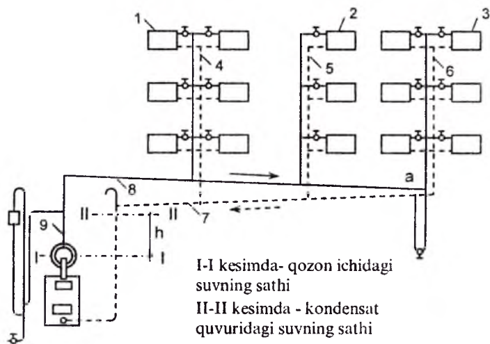
9.2-rasm. Quyidan taqsimlanuvchi va quruq kondensat quvurli bug'li isitish tizimining prinsiplial sxemasi
