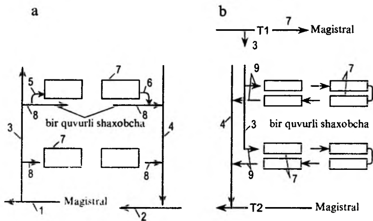
5.2-rasm Pastdan (a) va yuqoridan (b) uzatuvchi suvli gorizontal isitish tizimlari: 1, 2 – uzatuvchi va qaytaruvchi magistral; 3 va 4 – uzatuvchi va qaytaruvchi tirgak; 5 va 6 – uzatuvchi va qaytaruvchi ulama; 7 – isitish asboblari; 8 – bir quvurli shaxobcha; 9 – bifilyar tarmoq
