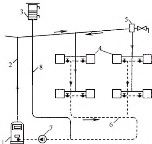
1.4-rasm. Sun'iy harakatlanuvchi yuqoridan taqsimlanuvchi ikki quvurli suvli isitish tizimining prinsipial sxemasi: 1 – issiq almashtirgich ( teploobmeni ); 2 – tirgak; 3 – kengaytiruvchi sig'im; 4 – isitish asbobi; 5 – havo jo'mragi; 6 – qaytaruvchi magistral nasos quvuri; 7 – uyurmaviy nasos; 8 – kengaytiruvchi idishning tutashtiruvchi quvuri
