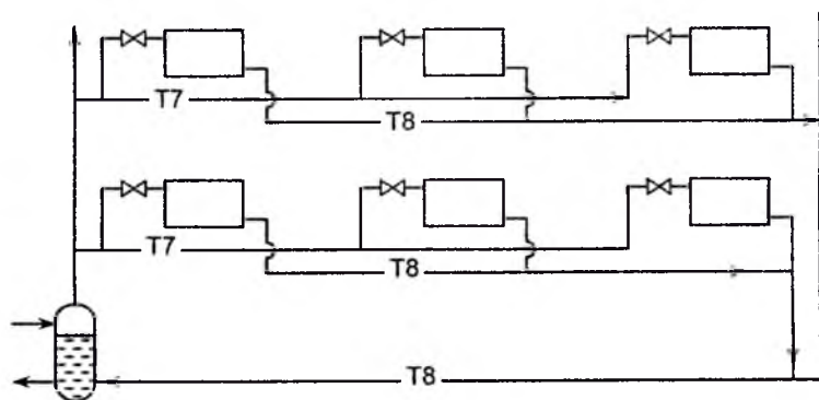
15.4-rasm. Gorizonttal ikki quvurli past haroratli bug'li isitish tizimining umumiy ko'rinishi
