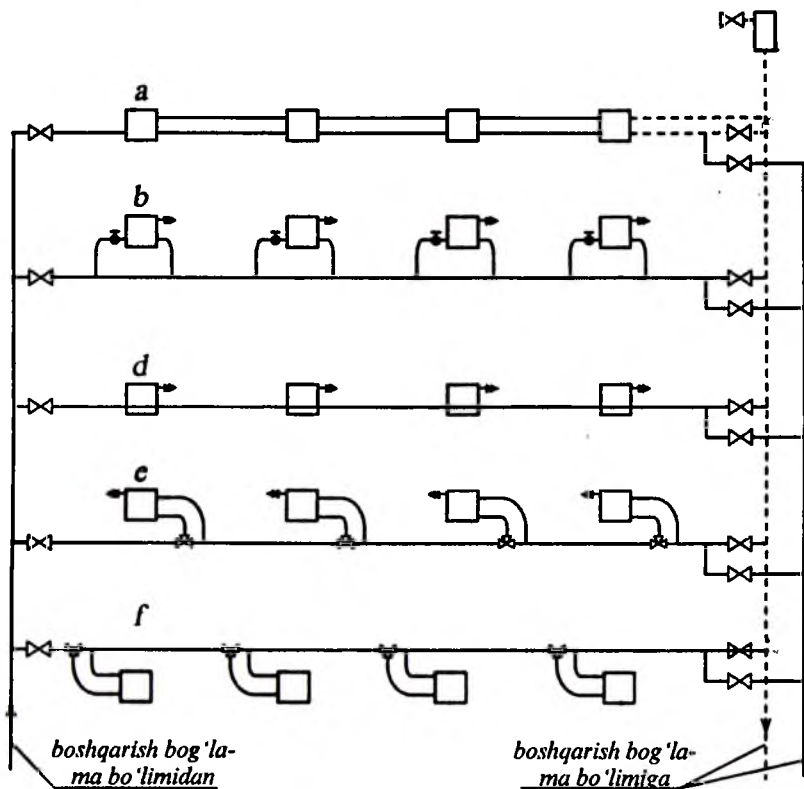
1.6-rasm. Sun'iy harakatlanuvchi suv bosimi ta'sirida ishlaydigan bir quvurli gorizontaal isitish tizimlarining prinsipial sxemasi: a) issiq suvni to'g'ridan-to'g'ri to'liq miqdorda isitish asbobi orqali o'tish uslubi; b) birlashtiruvchi uzatma orqali isitish asboblarning ulanish uslubi; d) to'g'ridan-to'g'ri isitish asbobiga ulanish uslubi; e) boshqariluvchi, to'g'ridan-to'g'ri plintusgardishli ulash uslubi; f) to'g'ridan-to'g'ri, boshqariluvchi, deraza tagiga ulanuvchi gorizontaal o'rnatilgan isitish asboblari
