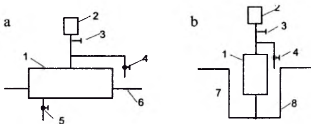
5.20 - rasm. Havo yig'uvchi uskunalar va vantuzlarning o'rnatilishi: 1 - havo yig'uvchi moslama; 2 - vantuz; 3 - ta'mirlash va taftish davrida ishlatiladigan vantuzning jo'mraki; 4 - qo'l bilan ishlatiladigan jo'mrak; 5 - havo yig'uvchi moslamaning suv chiqaruvchi quvuri; 6 - magistral quvur; 7 - havo harakati yo'li; 8 - sirtmoq shaklidagi quvur
