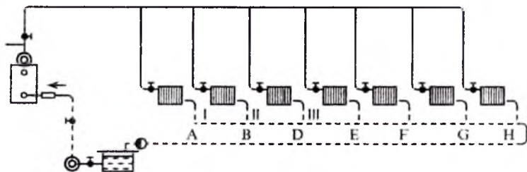
9.7-rasm. Kondensat va magistral bug' quvurlarining halqali harakatda bo'lgan ikki quvurli isitish tizimining sxemasi: 1 – bug'dan ajralavotgan suv kondensatini ajratuvchi uskuna; 2 – bug' bosimini pasaytiruvchi uskuna; 3 – ortiqcha bosim ta'sirini kamaytiruvchi moslama; 4 – tarqatuvchi kollektor; 5 – bug' miqdorini boshqaruvchi jo'mrak; 6 – kondensat ajratuvchi uskuna; 7 – kondensat idishi; 8 – havo quvuri; 9 – kondensat nasos; x – siljimas tirgak
