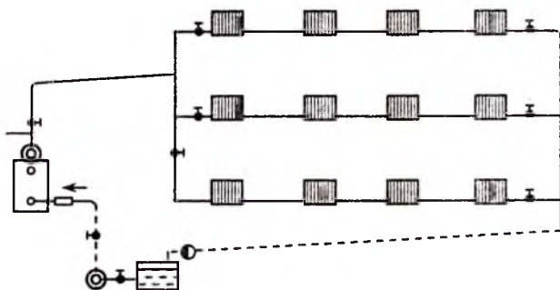
9.9-rasm. Bir quvurli gorizontaal joylashgan to'liq to'g'ri harakatli va yo'lma-yo'lakay bug' kondensat harakati ta'sirida ishlaydigan bug'li isitish tizimining sxemasi
