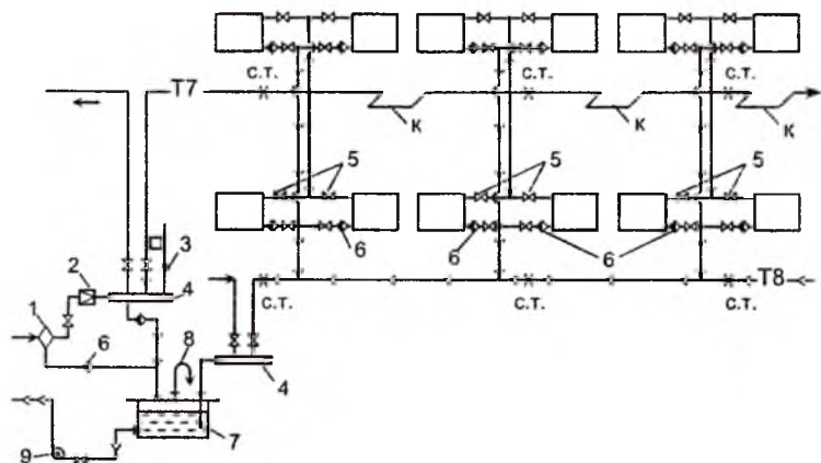
9.7-rasm. Kondensat va magistral bug' quvurlarining halqali harakatda bo'lgan ikki quvurli isitish tizimining sxemasi: 1 – bug'dan ajralavotgan suv kondensatini ajratuvchi uskuna; 2 – bug' bosimini pasaytiruvchi uskuna; 3 – ortiqcha bosim ta'sirini kamaytiruvchi moslama; 4 – tarqatuvchi kollektor; 5 – bug' miqdorini boshqaruvchi jo'mrak; 6 – kondensat ajratuvchi uskuna; 7 – kondensat idishi; 8 – havo quvuri; 9 – kondensat nasos; x – siljimas tirgak
