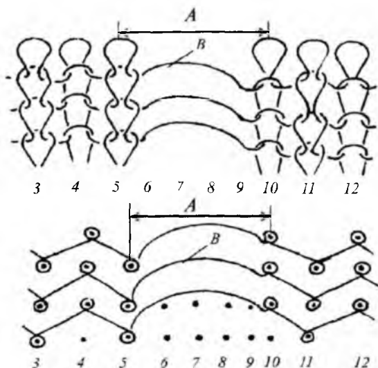
4.37.3-rasm. To'liq bo'lmagan ribana o'rilishli to'qimaning tuzilishi va grafik chizmasi.
