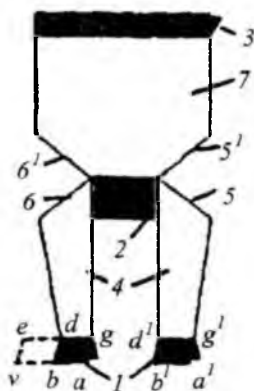
7.5-rasm. JET-2F mashinasida olinadigan sviterning yoymasi.
