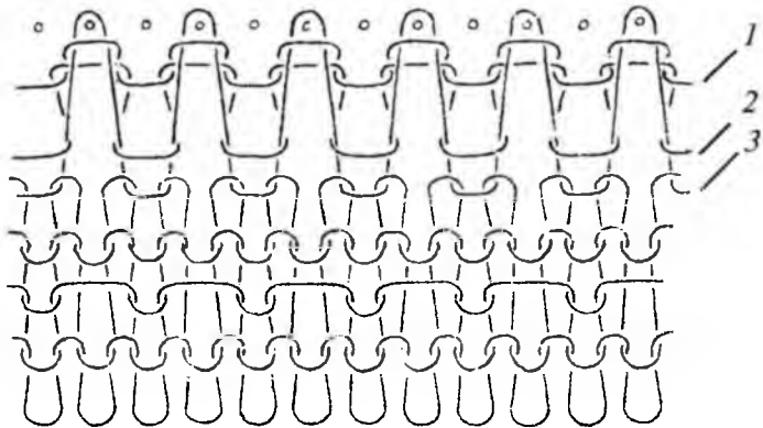
2.8-rasm. Ripshaybasiz, aylana ignadonli to'quv avtomatida to'qilgan paypoqning birlashtiruvchi chokini platinalar yordamida hosil qilish (platinalar yordamida tikish).
