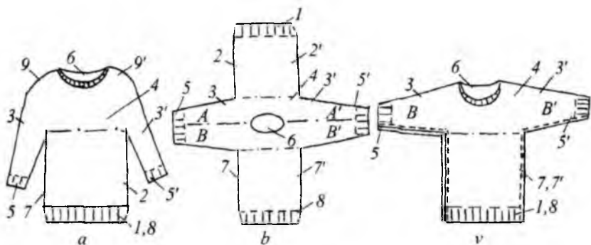
7.7-rasm. Yarim muntazam usulda ishlab chiqarilgan ustki trikotaj mahsulotlarining tuzilishi.
