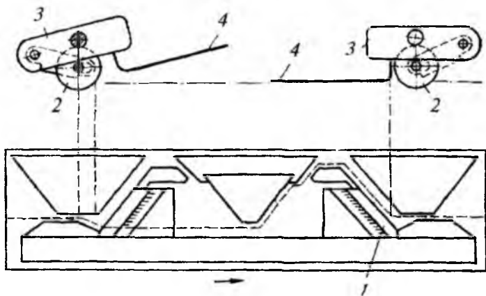
2.27-rasm. Halqa qatorlarini ignadon oralig'iga yo'naltiruvchi (tortuvchi) chivikli qurilma tuzilishi.
