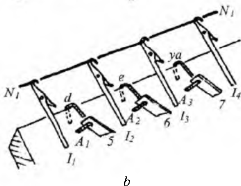
7.12-rasm. G'ilof va poyandozning dastlabki qatorini to'qish jarayoni: a – arqoq ipini ignalar oralig'iga joylashtirish jarayoni; b – to'quv ignalarga yangi ipni joylashtirish jarayoni.
