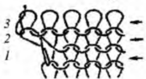
4.10-rasm. Halqalarni qo'shish va qo'shilgan ignalarga halqaning yarim yoyini kiygizish usuli bilan hosil qilingan gardish tuzilishi.
