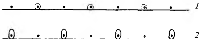
4.36-rasm. Hosilali suprem to'qimani to'qishdagi grafik chizmasi.
