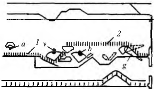
5.3-rasm. Ishlayotgan kichik tovonchali ignalarni igna zulllarida o'ngdan chapga harakatlanish sxemasi: a – ignalarni qo'shuvchi qurilma; b , v – ishlayotgan ignalar sonini qisqartiruvchi qurilma; g – tovon zulfi.
