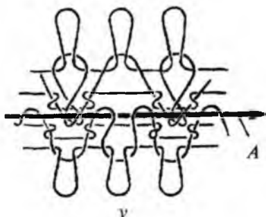
6.3-rasm. Paypoqning yopiq uch qismini birlashtiruvchi ip bilan hosil qilish sxemasi.
