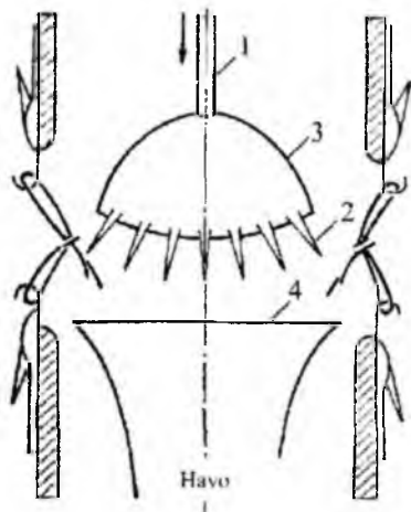
2.35-rasm. Zontikli taroqchali ignalar yordamida halqalarni tortish sxemasi.
