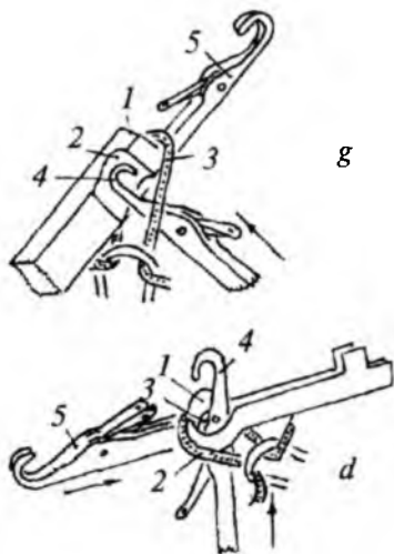
4.21g, d-rasm. Halqa ko'chirishda asosi «a» o'yoqli va ikki boshli juft tilchali ignalardagi halqalarni bir ignadon ignasidan ikkinchi ignadon ignasiga ko'chirish jarayoni.
