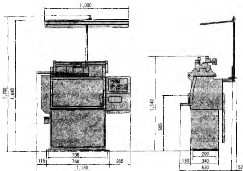
8.1-rasm. Qo'لقop to'quv avtomatining umumiy ko'rinishi.
