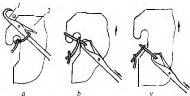
2.32-rasm. Yassi ignadonli fang qo'loq to'qiydigan avtomatlarda boshlang'ich halqa qatorlarini platinalar bilan hosil qilish sxemasi.
