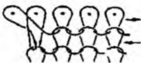
4.9-Rasm. Halqalarni igna yarim yoyini yangi ishga tushirilgan ignalarga ko'chirish (kengaytirish) yo'li bilan hosil etilgan gardish tuzilishi.
