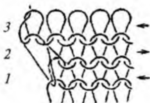
4.9-Rasm. Halqalarni igna yarim yoyini yangi ishga tushirilgan ignalarga ko'chirish (kengaytirish) yo'li bilan hosil etilgan gardish tuzilishi.
