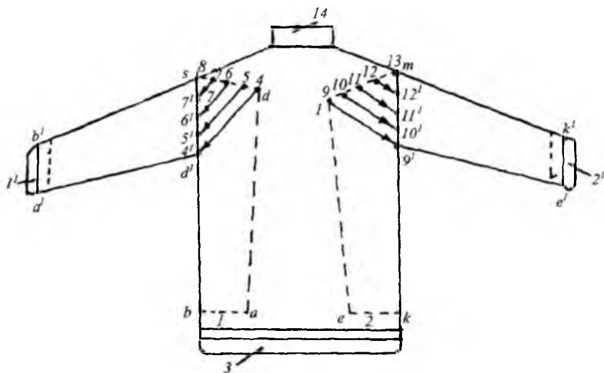
7.8-rasm. Yassi fang avtomatida jempnerni bir yo'la to'qish sxemasi.
