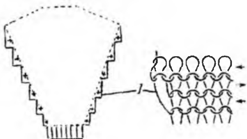
4.8-rasm. Chetdan igna qo'shish usulida hosil qilingan mahsulot gardishining tuzilishi.
