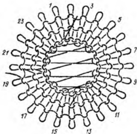
6.4-rasm. Yopiq qism tuzilishining sxemasi.
