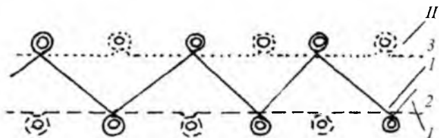
4.37.1.v-rasm. Murakkab aralash o'rilishli to'qimaning grafik chizmasi: 1 – ribana o'rilishli qator; 2, 3 – to'liq bo'lmagan suprem o'rilishli qator.
