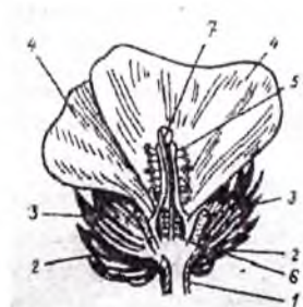
4—rasm. G‘o‘za gulining ko‘ndalang kesimi: 1-gul bandi; 2-shona barg; 3-gul kosa; 4-gul tojibarg; 5-changchi; 6-tuguncha; 7-urug‘cha tumshuqchasi.
