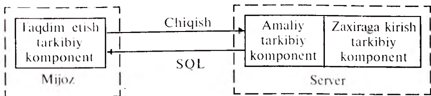
10.5-rasm. Ma'lumotlar bazasining serverli modeli.
