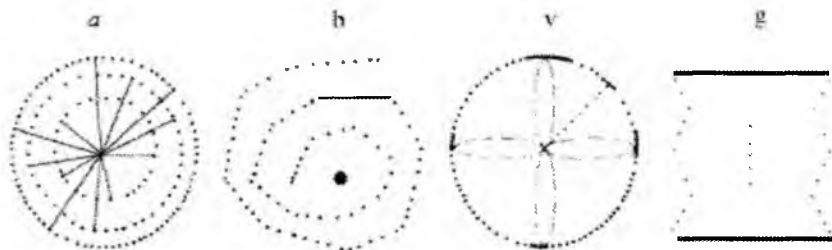
2.11-rasm. Elektron-blokli taxeometriyada piket nuqtalari syomkasining sxemalari: a –radius bo'yicha; b –spiral bo'yicha; v –nurli; g –zigzagli (siniq chiziqli)
