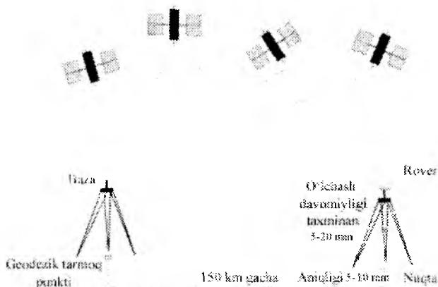
3.9-rasm. Tezkor statika usuli
