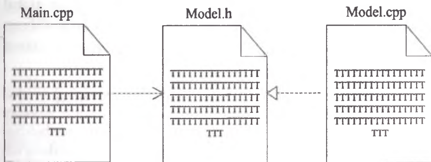
7.16-rasm. C++ bajariladigan faylni komponentlash diagrammasining namunasi.
