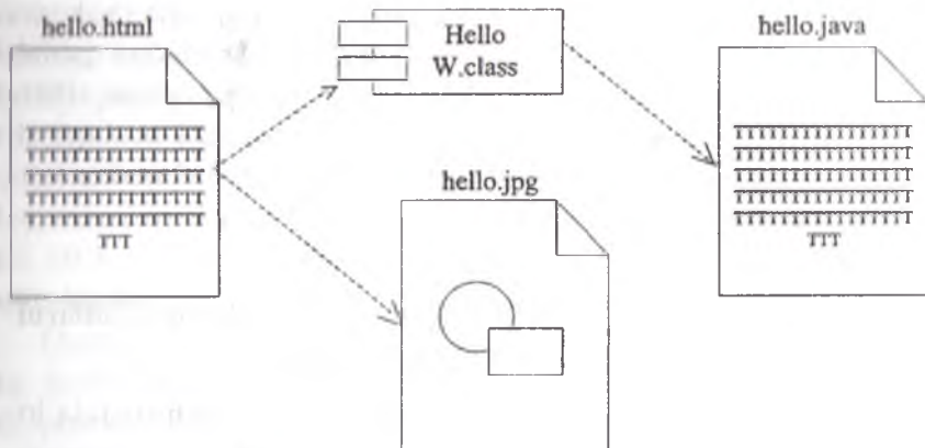
7.15-rasm. «Hello World» matni va fotosuratini chiqaruvchi internet-ilova komponentlash diagrammasi.
