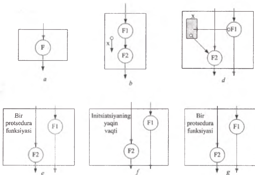
2.1-rasm. Modullar aloqadorligi: a – funksional; b – ketma-ket; d – axborot; e – protsedurali; f – muvaqqat; g – mantiqiy
