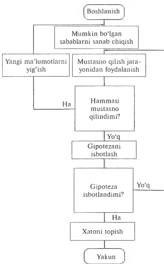
10.4-rasm. Deduksiya usuli bilan sozlash jarayonining sxemasi.
