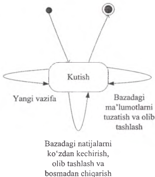
8.8-rasm. Kombinatorli-optimallashtirilgan masalalarni yechish tizimining abstrakt dialog grafiği.
