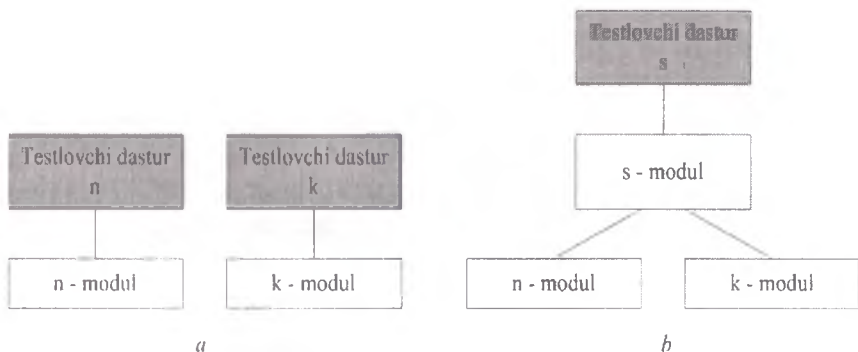
9.2-rasm. Yuqorilovchi yondashuvda dasturiy ta'minotni testlash: a – quyi darajadagi avtonom testlash; b – navbatdagi darajadagi testlash.
