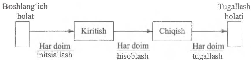
4.4-rasm. Atrof-muhit bilan o'zaro faol harakatlanmaydigan dasturiy ta'minot holatining o'tish diagrammasi.
