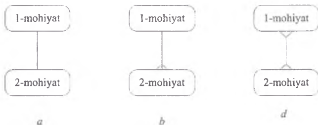
4.22-rasm. Barker notatsiyasida munosabatlarning belgilanishi: a – «bittaga-bitta»; b – «bitta-ko'pga»; d – «ko'p-ko'pga».
