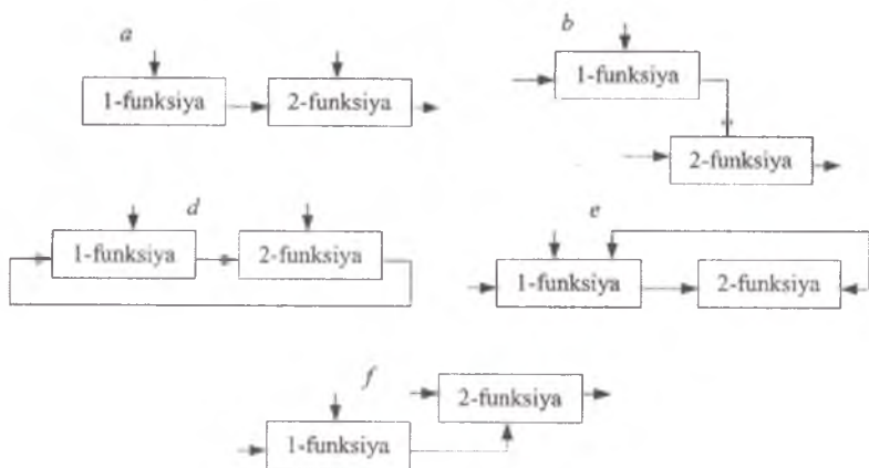
4.7-rasm. Bloklarning ta'sir turlari: a – kirish; b – boshqaruv; d – kirish bo'yicha qayta aloqa; e – boshqaruv bo'yicha qayta aloqa; f – chiqish ijrochi.
