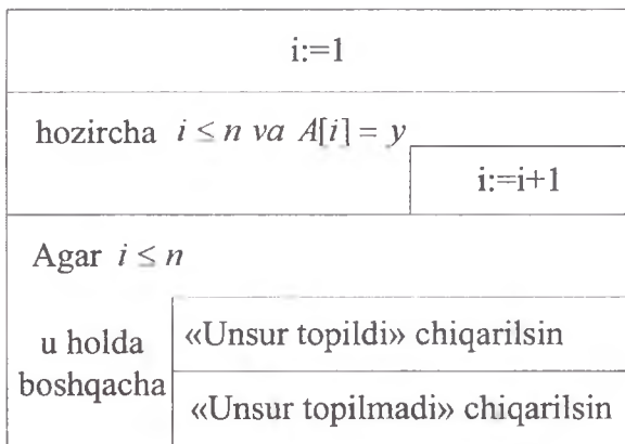
2.5-rasm. Izlash sikli algoritmi.
