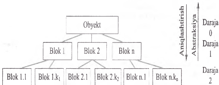
1.8-rasm. Blokli-iyerarxiyali yondashuvdagi bloklarning tavsifidagi mavhumlik va aniqlik munosabati.
