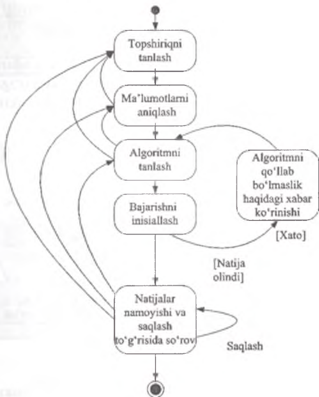
8.10-rasm. Kombinatsiyalashgan turdagi abstrakt dialog grafi.
