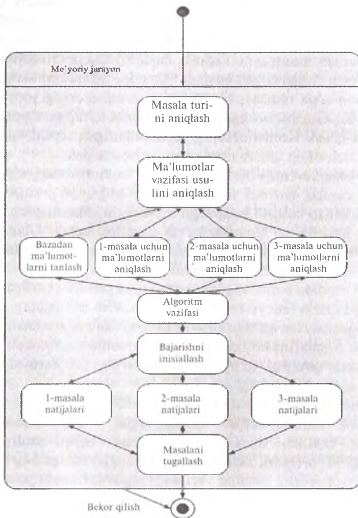
8.13-rasm. Yangi topshiriqning yangidan tuzilgan dialogi holati diagrammasi.
