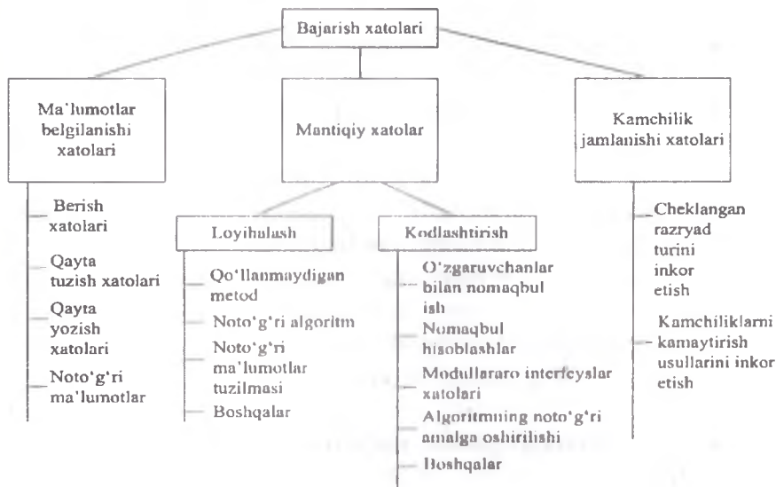
10.2-rasm. Ehtimolli sabablar bo'yicha bajarish bosqichi xatolarining tasnifi.
