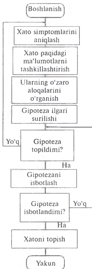
10.3-rasm. Induksiya usuli bilan sozlash jarayoni sxemasi.
