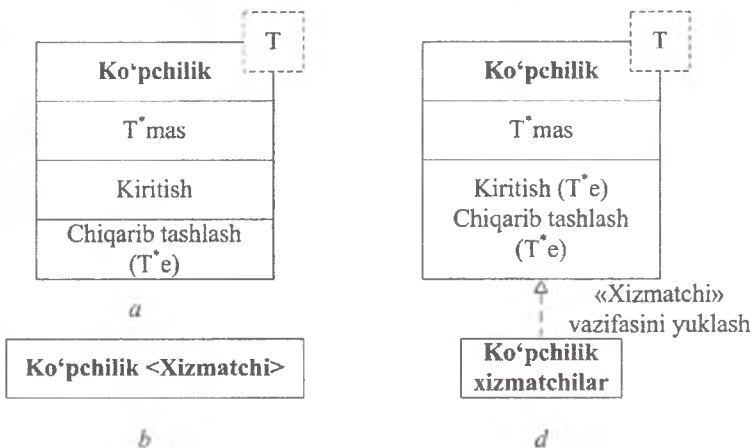
7.6-rasm. UML da interfeysning shartli belgilari:
