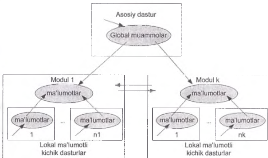
1.5-rasm. Modullardan tashkil topgan dasturlar arxitekturasini.
