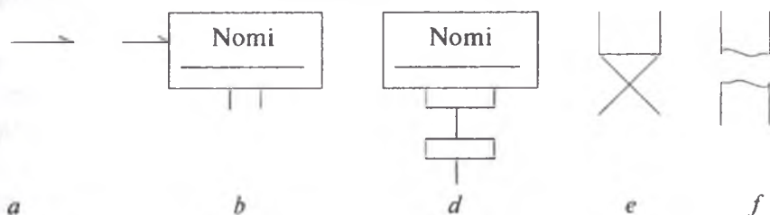
7.4-rasm. Boshqaruvni asinxron uzatishning shartli belgilari: a – asinxron xabar; b – obyektni yaratish (asinxron bo'lishi shart emas); d – obyektni faollashtirish; e – obyektni yo'q qilish; f – bo'linish (boshqa ishlanmalarni bajarish).
