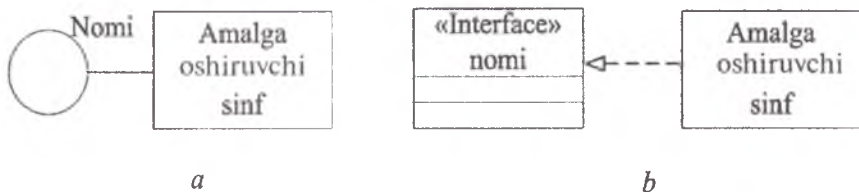
7.8-rasm. Interfeysni amalga oshirishning shartli belgilari: a – siyiq shakl; b – amalga oshirish munosabati ko‘rsatilgan shakl.
