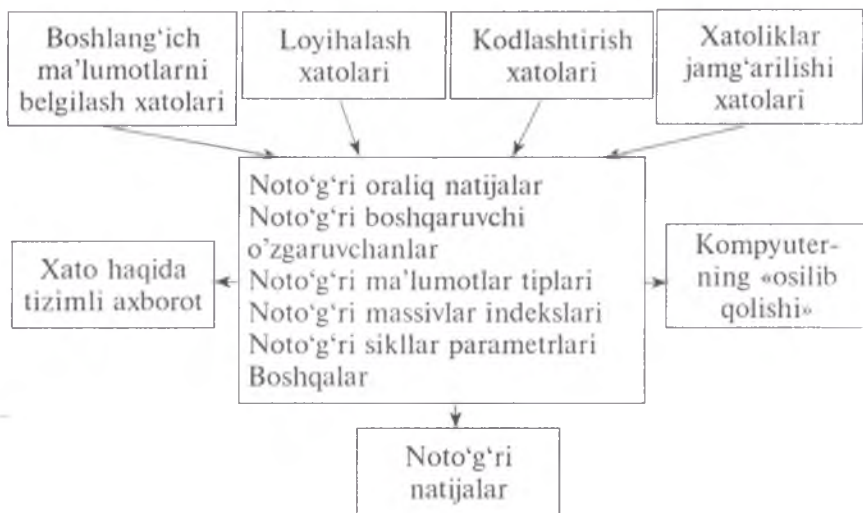
2.7-rasm. Xatolar namoyon bo'lish usullari.
