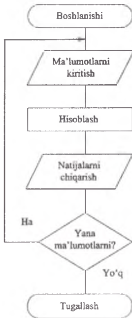
8.3-rasm. Sodda interfeysga ega dastur algoritmining tipik tuzilmasi: a – ketma-ket; b – takrorlash imkoniyati bilan.
