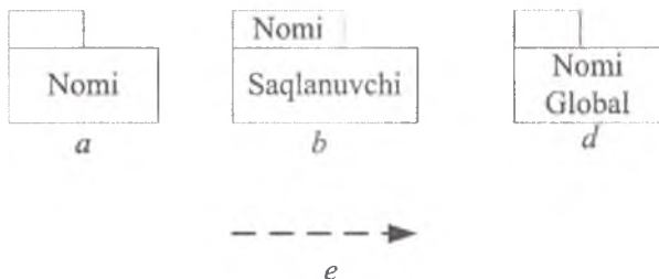
7.2-rasm. Paketlar diagrammasi qo'llaniladigan shartli belgilar: a – paket; b – mavjud ma'lumotlar belgilangan paket; d – global paket; e – sinflar bog'liqligi (yoy chaqiruvlar yo'nalishini ko'rsatadi).
