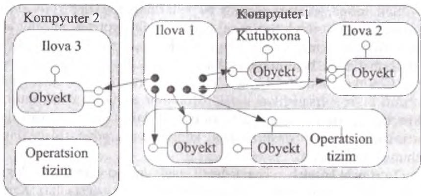
1.7-rasm. Turli xildagi dasturiy komponentlarning o‘zaro ta’siri.
