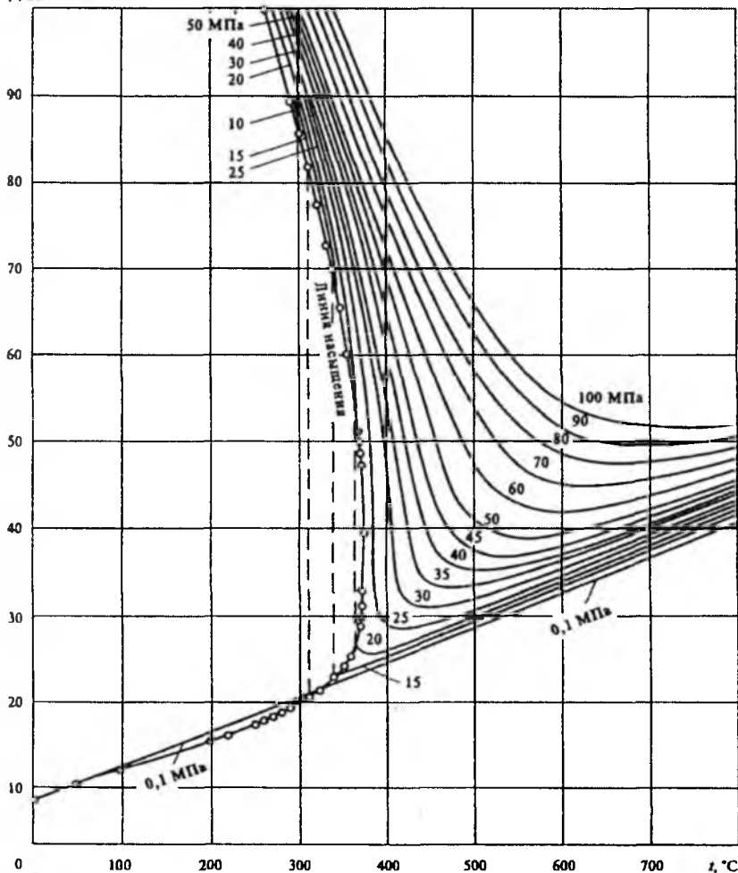
3-рasm. Suv va suv bug'larining dinamik qotishqoqligi harorat va bosim koeffitsiyentiga bog'liqligi
