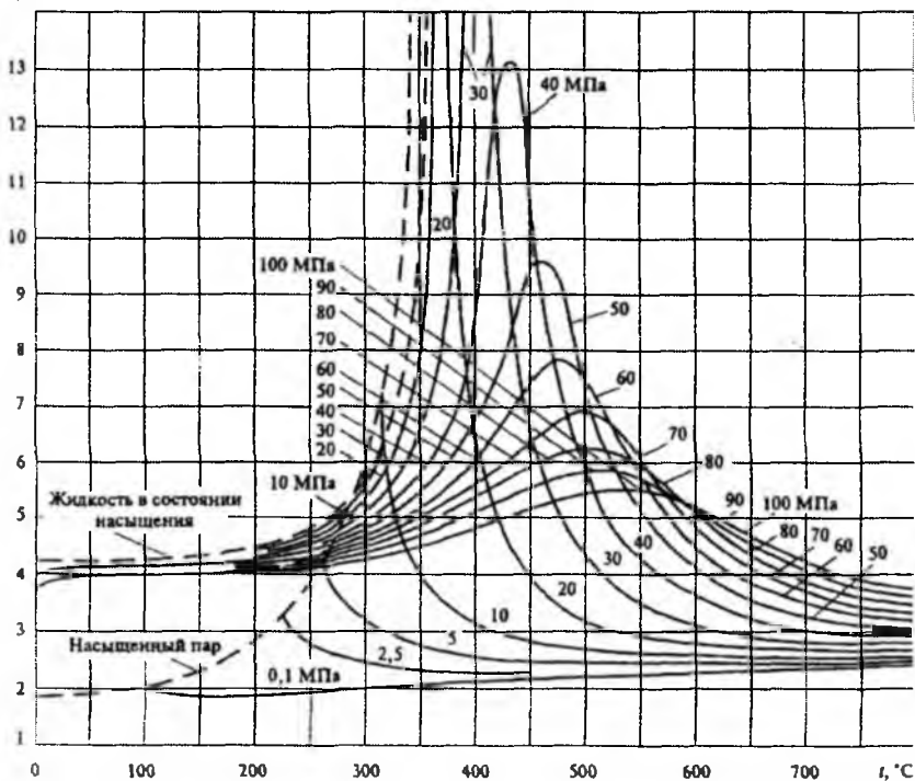
2-рasm. Suv va suv bug'larining isobarik issiqlik sig'ining harorat va bosimga bog'liqligi
