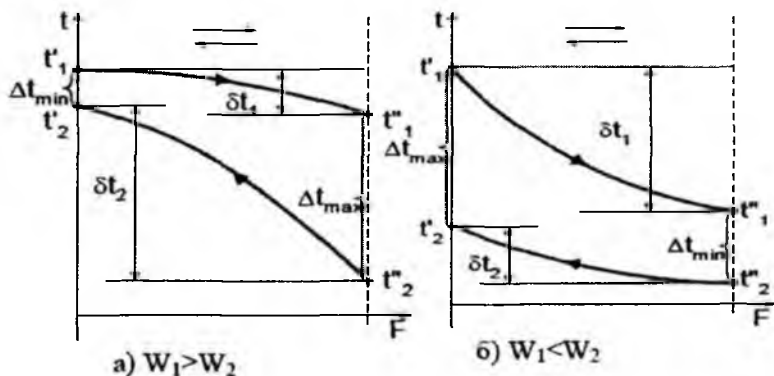
2.2 b-rasm. Issiqlik tashuvchilarning oqimga qarshi harakatlanish sxemasida ularning suv ekvivalentlari nisbatiga bog'liq ravishda qaynoq va sovuq issiqlik tashuvchilar haroratining issiqlik almashinish yuzasi bo'ylab o'zgarishi
