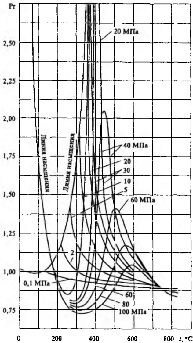
5- рasm. Prandtл сув va сув bug'и miqdorini harorat va bosimga bog'liqligi
