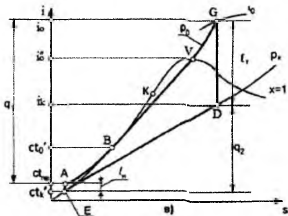
1.13-rasm. Bug'ni ortiqcha qizitish bilan kechadigan Renkin sikli
