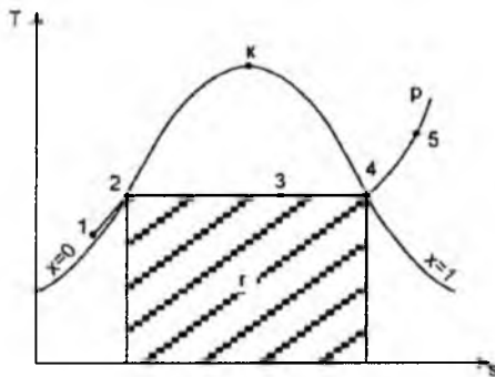
2.1-rasm. Suv bug‘ining fazaviy T, s - diagrammasi
