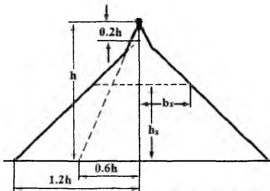
8.7- rasn. Trosli yashin qaytargichning himoyalash sohasi.
