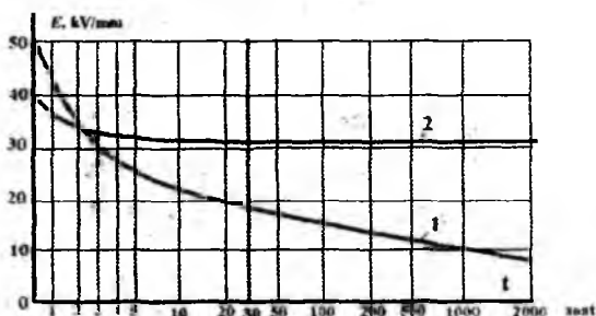
4.16- rasm. Qovushoq moy singdirilgan (1) va moy to'ldirilgan (2) kabellarning teshilish mustahkamligining kuchlanishning ta'sir etish vaqtiga bog'liqligi.
