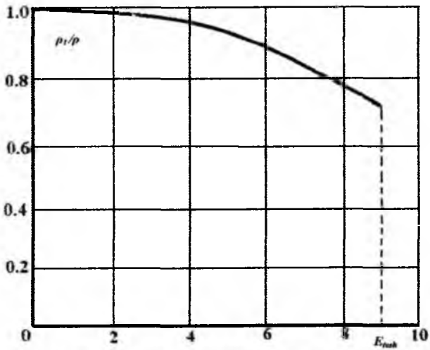
8.13- rasm. Tuproqning solishtirma qarshituvini elektr maydon kuchlanganligiga bog'liqligi \frac{\rho_1}{\rho} = f(E) .
