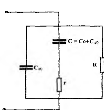
6.2- rasm. Izolyatsiyaning almashtirish sxemasi.
