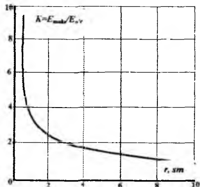
2.1- rasm. Silindrik kondensatorning tashqi radiusi 10 sm va o'zgaras bo'lganda bir jinsli bo'lmaganlik koeffitsienti K ning silindrning ichk radiusi r ga bog'laqligi.
