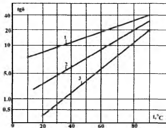
6.6- rasm. Transformatorlar izolyatsiyasi uchun \text{tg } \delta = f(t^\circ) funksional bog'lanishlarning grafigi: 1 va 2 – ho'llangan holatlar; 3 – quruq holat.
