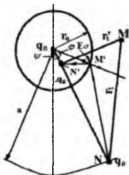
4.10- rasm. Parchalangan o'tkazgichlar elektr maydon kuchlanganligining taqsimlanishini hisoblashga doir.
