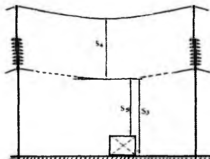
4.2- rasm. Portal rusmidagi tayanchda bajarilgan liniyaning izolyatsiya oraliqlarining ko'rinishi.
