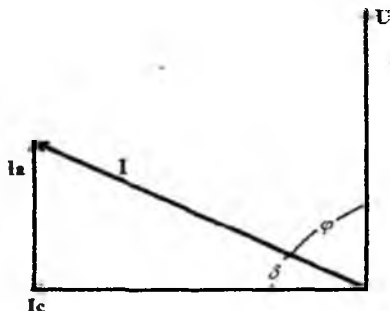
6.3- rasm. Sanoat chastotasidagi kuchlanish ostidagi izolyatsiyada tok va kuchlanishning vektor diagrammasi.
