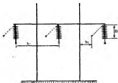
4.1- rasm. Portal rusmidagi tayanchda bajarilgan liniyaning izolyatsiya oraliqlarining ko'rinishi.
