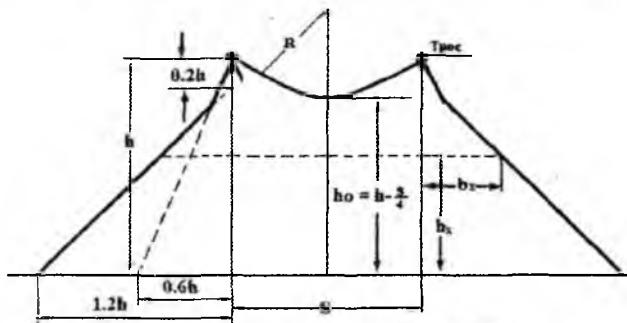
8.8- rasn. Ikkita trosning himoyalash sohasi.
