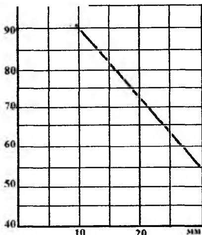
3.3- rasm. Chinningning 50 Gts chastotali o'zgaruvchan kuchlanishli bir jinsli bo'lgan maydonda hisobiy elektrik mustahkamligi
