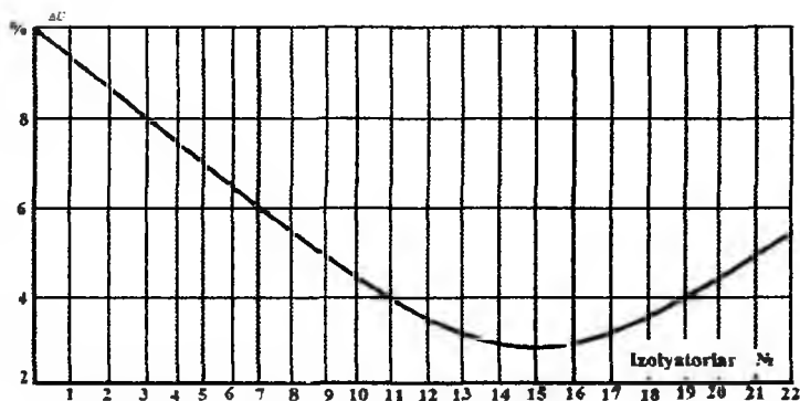
4.7- rasmlar. Kuchlanishi 500 kV bo'lgan IIC-12 rusmli tutib turuvchi izolyatorlar shodasi bo'ylab kuchlanishning taqsimlanishi (shodadagi umumiy kuchlanishga nisbatan foizlarda).
