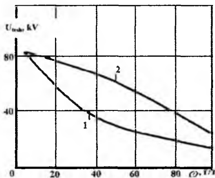
3.5-rasm. Atrof muhit temperaturasi 25^{\circ}\text{S} va 50 Gts da transformator moyining teshilish kuchlanishini namlikka bog'liqligi: 1 – tarkibida 50 g/t konsentratsiyali qattiq birkmalar mavjud bo'lgan texnik toza moy uchun; 2 – tarkibida 0,5 g/t konsentratsiyali qattiq birkmalar mavjud bo'lgan texnik toza moy uchun.
