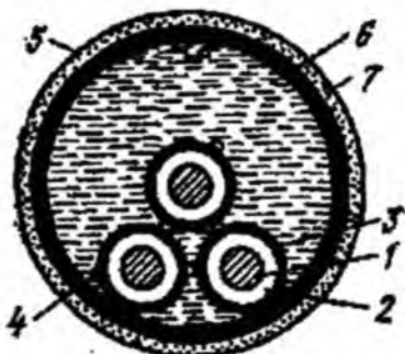
4.19- rasm. Bosim ostida moy to'ldirilgan quvurda joylashgan kabel: 1- pay; 2- izolyatsiya; 3- zichlaydigan (germetik) yopqich; 4 - yarim aylana o'tkazgich; 5 - po'lat quvur; 6- moy; 7- zanglashga qarshi yopqich qatlam.
