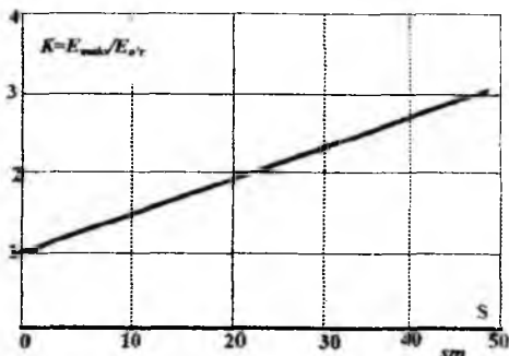
2.2- rasm. Diametri 20 sm bo'lgan sharlar orasidagi elektr maydon bir jinsli o'lmaganlik koeffitsientining sharlar orasidagi masofaga bog'liqligi.
