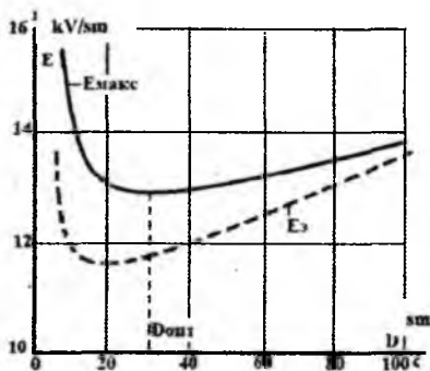
1.8- rasml. Parchalangan o'tkazgich sirtidagi maksimal va ekvivalent elektr yurituvchi kuchning o'tkazgichlar orasidagi masofaga bog'liqligi.
