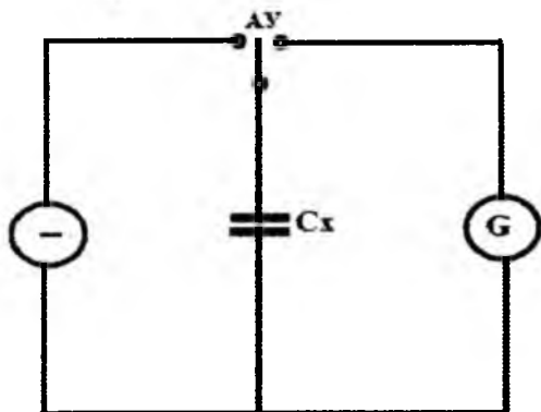
6.5- rasm. Ikkita chastotada izolyatsiyaning sig'imini o'lchashning prinsipl sxemasi.
