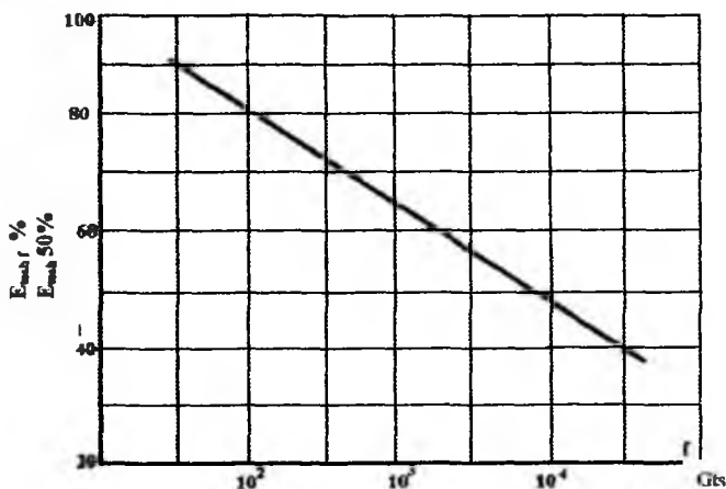
5.7- rasm. Qog'oz-moyli izolyatsiya elektrik mustahkamligining chastotaga bog'liqligi.
