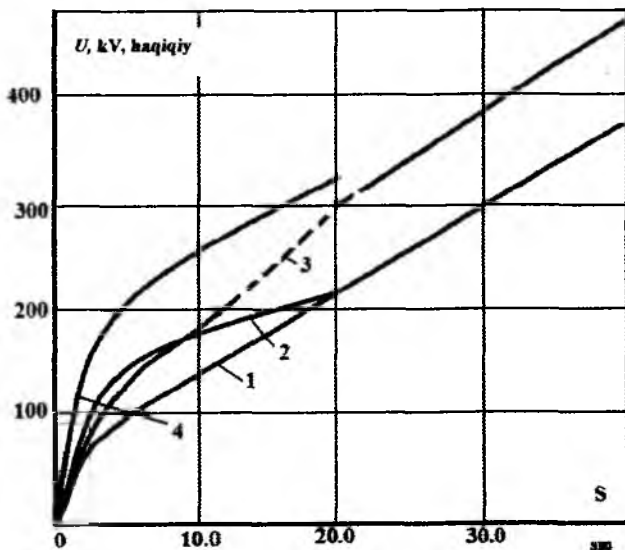
5.4- rasm. Sanoat chastotasida elektrodni yupqa qatlamli dielektrik bilan qoplanishining ta'siri. Elektrodlar parallel: 1 – diametri 3 mm qoplamasiz; 2 – diametri 10 mm qoplamasiz; 3 - diametri 3 mm ikki qavatli kabel qog'ozidan yasalgan qoplama o'rnatilgan; 4 – diametri 10 mm ikki qavatli kabel qog'ozidan yasalgan qoplama o'rnatilgan. Moyni norma bo'yicha elektrik mustahkamligi 26 – 28 kV ta'siri et 2,5/mm
