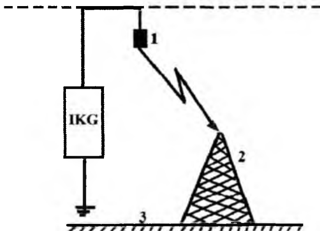
8.2- rasm. Yashin qaytargichning himoyalash sohasini tajribada aniqlash sxemasi.
