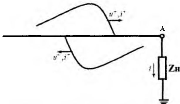
7.5- rasm. Tugunda sinayotgan to'liqni hisoblash uchun sxema.
