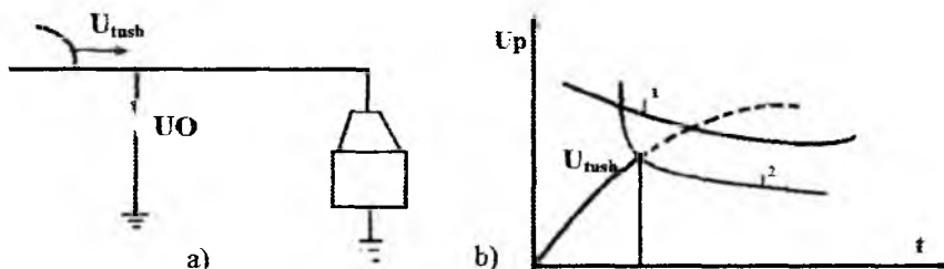
8.9- rasm. Himoya uskunasi ishlar prinsipi: a— uchqun oraligʻi (UO)ning sxemasi; b— himoyalananayotgan element (1) va uchqun oraligʻi (UO)ning volt—sekund xarakteristikalarini moslashtirish.
