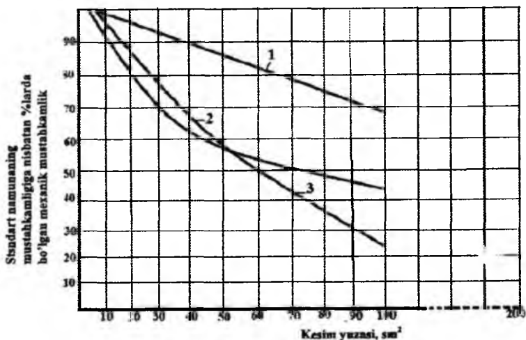
3.4- rasm. Silindr shaklidagi chinning mexanik mustahkamligini ko'ndalang kesim yuzasiga bog'liqligi: 1 – siqishga; 2 – cho'zishga; 3 – cgishga.
