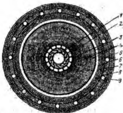
4.18- rasmda kuchlanishi 220 kVga mo'ljallangan o'rta bosimli kabel:
