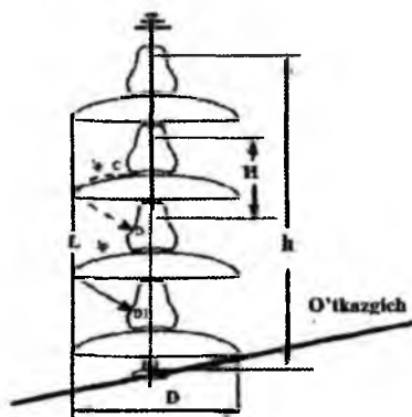
4.5- rasml. Osiluvchan izolyatorlar shodasining asosiy ulchamlari:
