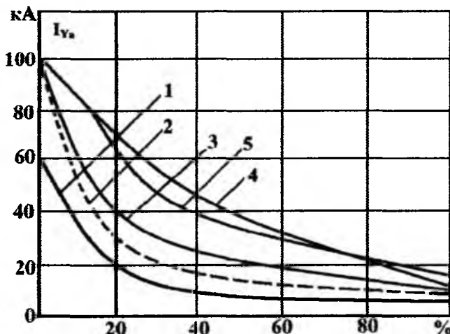
7.3- rasm. Turli manbalardan olingan yashin toki amplitudasining protsentlardagi egri chizig'i: 1- Amerikaning osmono'par binosidagi razryadlar; 2- Amerika injener – elektrklar institutining tavsiyasi asosida olingan ma'lumot; 3- Sobiq SSSRda qabul qilingan ma'lumot; 4 – Lyuis va Faustning ma'lumotlari bo'yicha; 5 – Amerikaning elektr uzatish liniyalarida oxirgi marta kuzatilgan tok amplitudasi.
