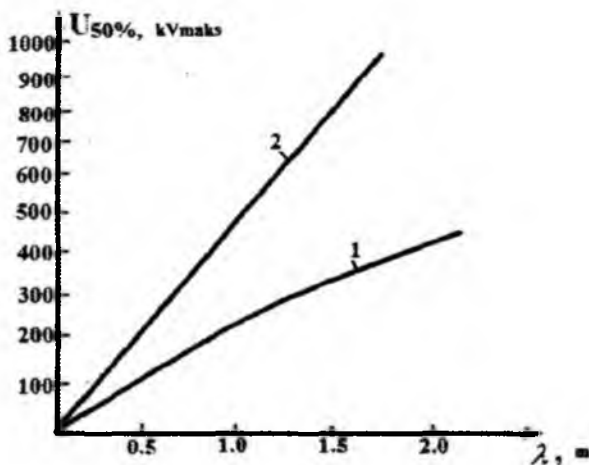
7.9- rasm. 50% li impuls razryadlanish kuchlanishining izolyatorlar shodasining uzunligiga bog'liqligi: 1 – IIM -4,5 rusmli izolyatorlar shodasi uchun; 2 – II-4,5 rusmli izolyatorlar shodasi uchun.
