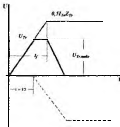
7.10- rasm. Tayanchlar oralig‘ining o‘rtasida trosqa yashin urilgandagi kuchlanish impulsi.
