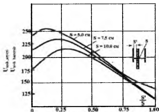
3.8-rasm. Sanoat chastotasi bilan (50 Gts) o‘zgaruvchan kuchlanishda bir jinsli bo‘lmagan maydonda transformator moyining teshilish kuchlanishiga yupqa to‘siqning ta’siri.
