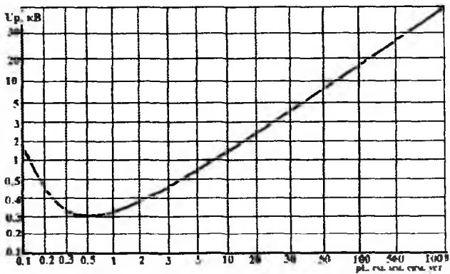
2.4- rasm. Bir jinsli elektr maydonida havo oralig'ini uchun Pashen egri chizig'i U_p = f(pL) .
