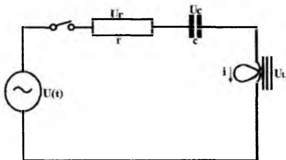
7.20- rasm. Nochiziqli induktivligi bo'lgan oddiy tebranish konturining prinsipl sxemasi
