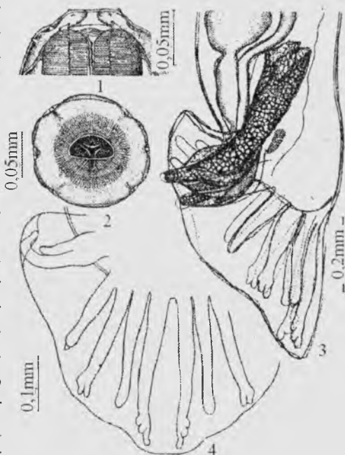
37-rasm. Diktiokaulalarning morfologiyasi. Dictyocaulus filaria (Rud., 1809) (Boev, 1952 buyincha): 1) boshi (yondan); 2) boshi (yukoridan); 3) erkak nusxantig dumi sikulalar bilan; 4) bursaning bir kismi.
