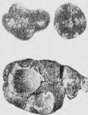
16-rasm. Senuroz pufaklar (yuqorida) bosh miyada joylashgan senuruslar
