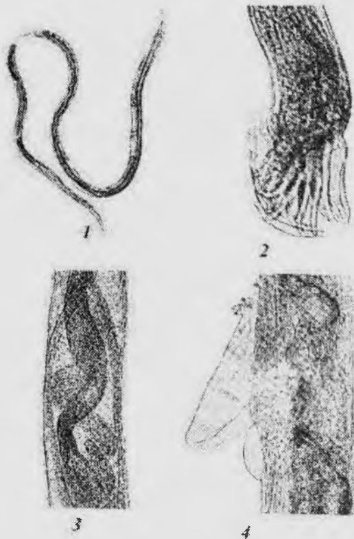
26-rasm. Mikrofoto preimaginal (voyaga yetmagan 20-22 kunlik) marshallagiyalar: 1) urg'ochi nusxaning umumiy ko'rinishi 2) erkak nusxaning jinsiy bursasi: 3 va 4) urg'ochi nusxa tanasining bachadon va jinsiy teshik (vulva) qismi. (Original)
