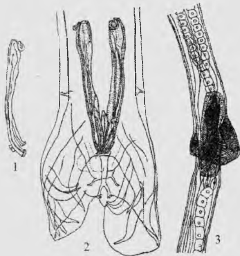
29-rasm. Ostertagiylarning morfologiyasi. Ostertagia (Ostertagia) ostertagi (Stiles, 1892): 1) spikula (Rensom, 1911 bo'yicha); 2) erkak nuxxaning dum qismi; 3) urg'ochisining jinsiy teshik (vulva) qismi (Travassos, 1921 bo'yicha)
