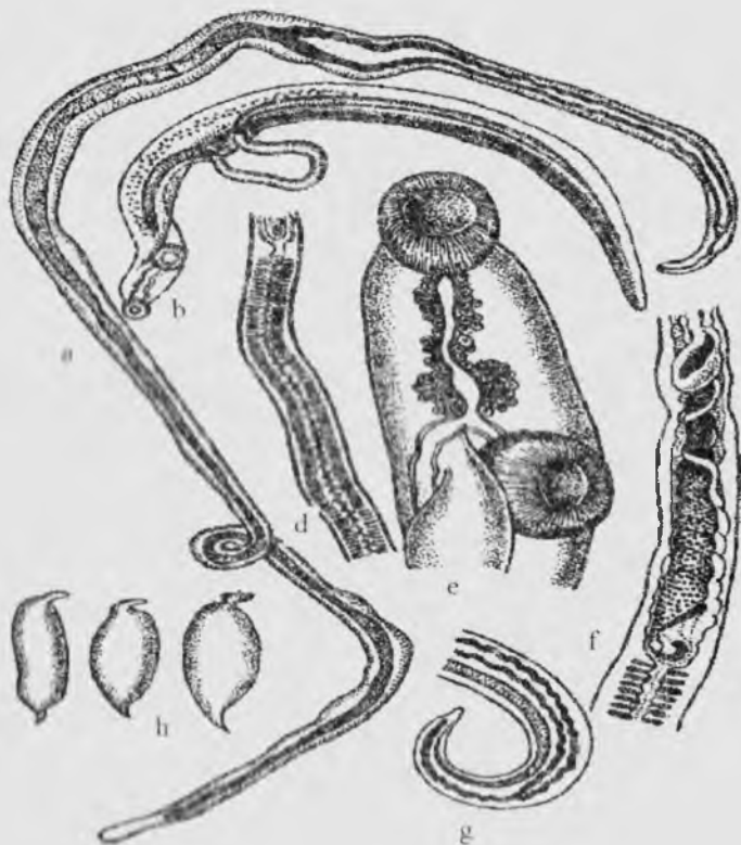
7-rasm. Orientobilgarziyalarning morfologiyasi Orientobilharzia turkestanica : a) erkak nusxasi; b) erkak va urgochi; d) urgochi nusxa tanasining bir qismi; e) tananing bosh qismi; f) urg'ochi nusxaning jinsiy apparati; g) erkak nusxaning dum qismi; h) tuxumlar (Ivashkin, Muxamadiev, 1981)
