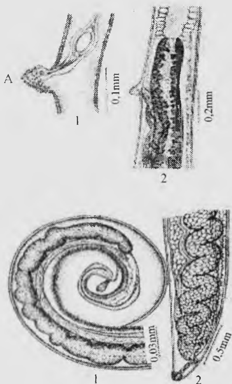
34-rasm. Trixotsefalyuslarning morfologiyasi: Trichotsefalus skrjabini (Baskakov, 1924), (Magomedbekov, 1953 bo'yicha). A) 1) urg'ochi nusxa vulvasidagi ilmoqchalar, 2) urg'ochi nusxaning vulva qismi. B) 1) erkak va 2) urg'ochi nusxaning orqa qismi va dum uchi.
