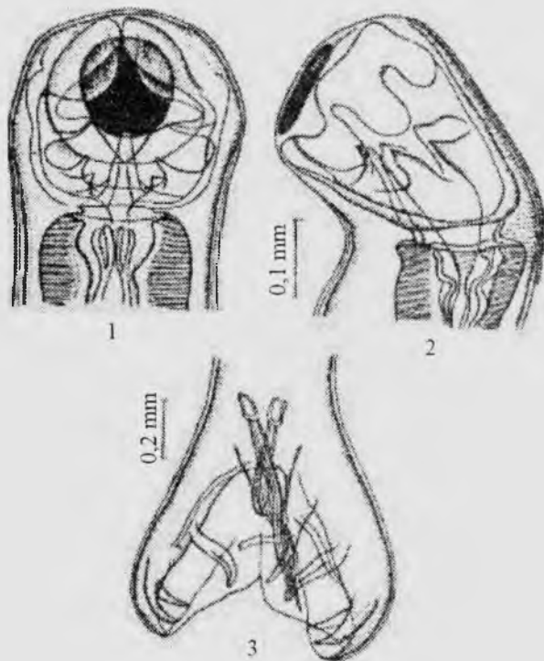
32-rasm. Bunostomlarning tuzilishi: 1-2) bosh qismi; 3) erkak bunostomlarning jinstiy bursasi (Skryabin va Shuls 1937)
