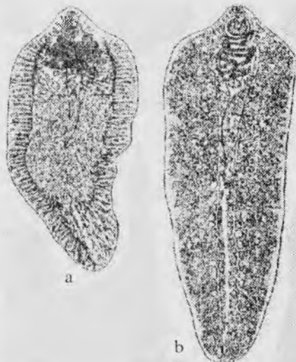
2-rasm. Fassiolalarning morfologiyasi. a) F. hepatica ; b) F. gigantica (Ivashkin, Muxamadiev, 1981)
