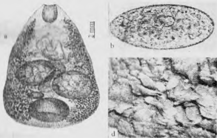
8 a -rasm. Paramfistomalarning morfologiyasi: a) Paramphistomum skrjabini (K Popov, 1936); b) paramfistomalarning tuxumi; c) paramfistomalar katta qorinda;
