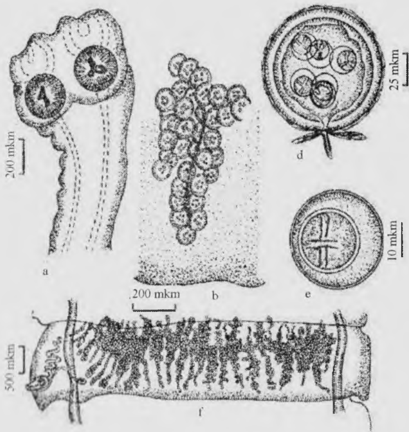
11-rasm. Tizanieziyalarning morfologiyasi. Thysaniezia giardi : a) skoleks; b) paruterin organ (tuxumdon)lar, d) yetilgan tuxumlari bor xaltacha, e) yetilgan tuxum; f) yetilgan bugin (Ivashkin, Muxamadiev, 1981)
