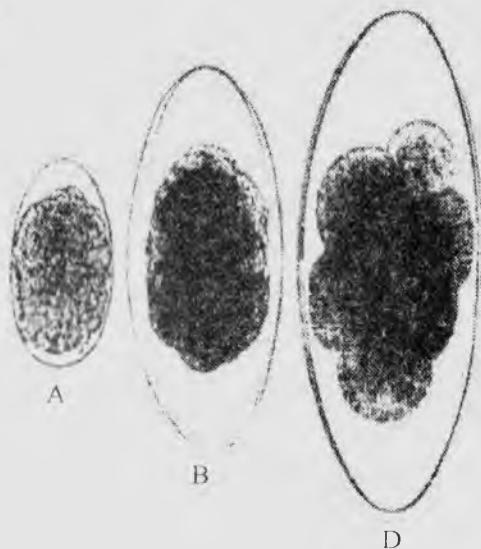
24-rasm. Strongilyatlarning tuxumlari: A) ko'pchilik strongilyatlarga (gemonx, ostertagiya, trixostrongilyus, kooperia, xabertna, bunostomum, ezofagostomum va boshq.); B) marshallagiya; D) nematodirus. (Original)
