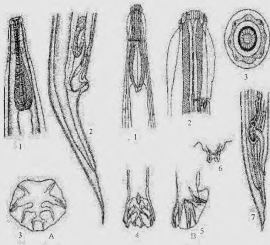
33-rasm. Ezofagostomlarning morfologiyasi: A) Oesophagostomum radiatum (Rudolphi, 1803) (Rensom, 1911 bo'yincha); 1) bosh qismi; 2) urgochisinning dum qismi; 3) erkak nusxaning bursasi. B) Oesophagostomum verulosum (Rud., 1809) (Gudey, 1924 buyincha) 1) va 2) tanasining bosh qismi; 3) boshining yukoridan ko'inishi; 4 va 5) erkak nusxaning dum qismi va bursasi; 6) jinsiy konus; 7) urgochisining dum qismi.
