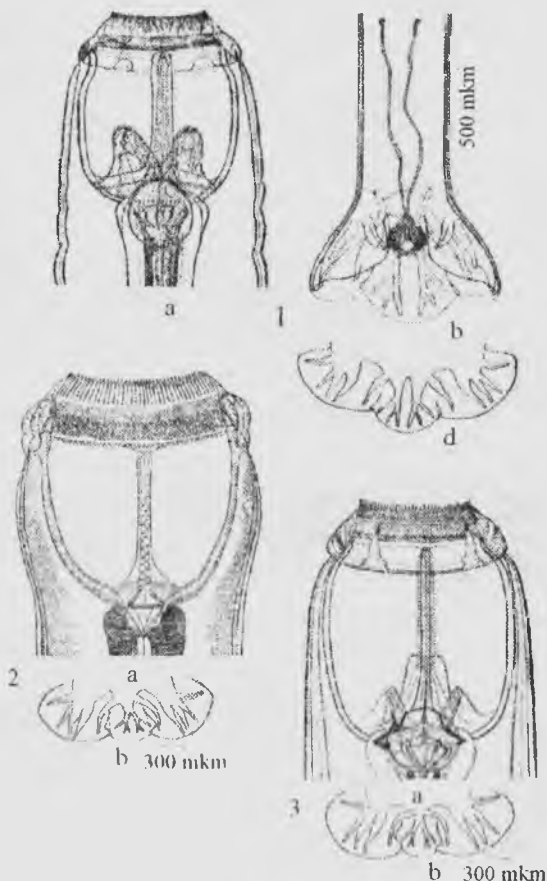
52-rasm. Strongilyatlarning morfologiyasi. (V.M.Ivashkin, G.M.Dvoynas, 1984): 1- Delaphondia vulgaris (a-og'iz kapsulasi b-erkak nusxasining dum qismi, b-kopulyativ bursa); 2- Alfortia edentatus (a- og'iz kapsulasi, b-kopulyativ bursa); 3- Strongylus equinus (a- og'iz kapsulasi, b-kapulyativ bursa).
