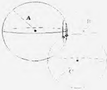
10.6.1-rasm. Trilateratsiy
