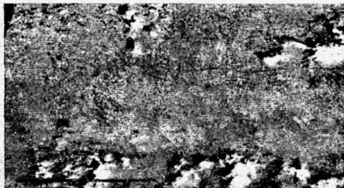
11.4.1.2–rasm. LANDSAT su'niy yo'ldoshi orqali 2009–yil aprel oyida Jizzax va Sirdaryo viloyatlari hududi bo'yicha olingan tasvirlar (V.X.Sherimbetov tomonidan keltirilgan materiallar).
