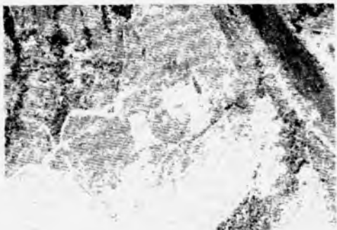
3.1.4-rasm. Aerofototasvir
