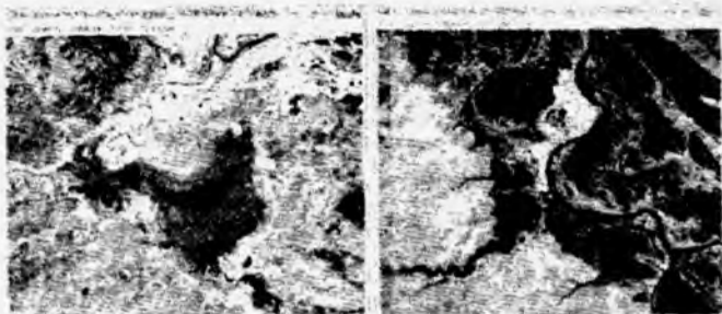
3.1.3-rasm. «LandSat» yerning su'niy yo'ldoshi yordamida olingan tasvir
