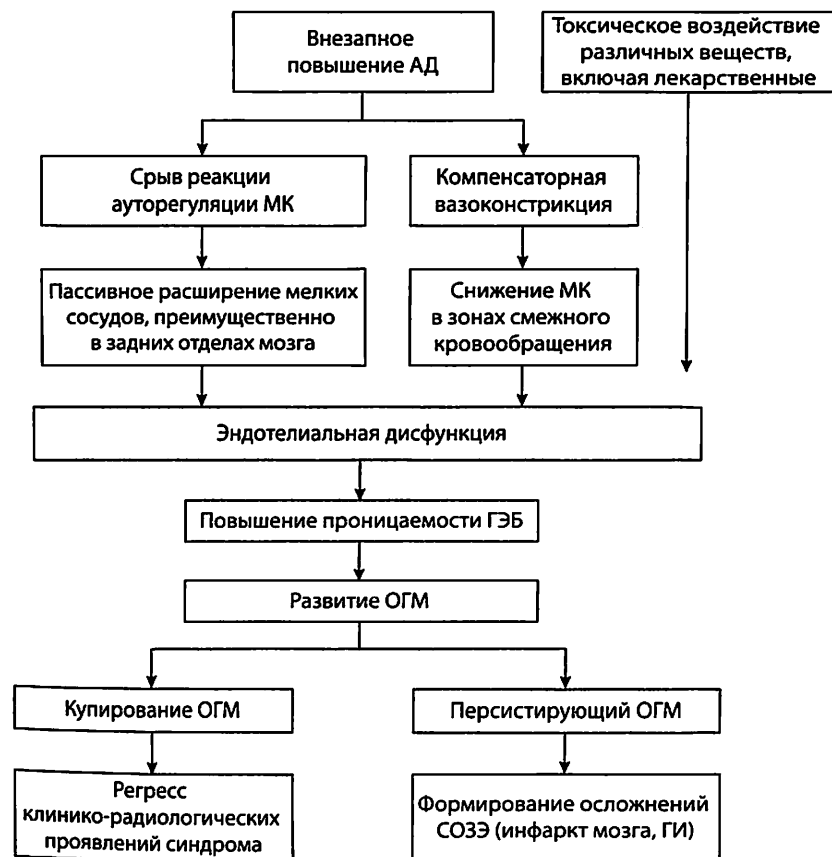
Рис. 5.1. Патогенез СОЗЭ.
