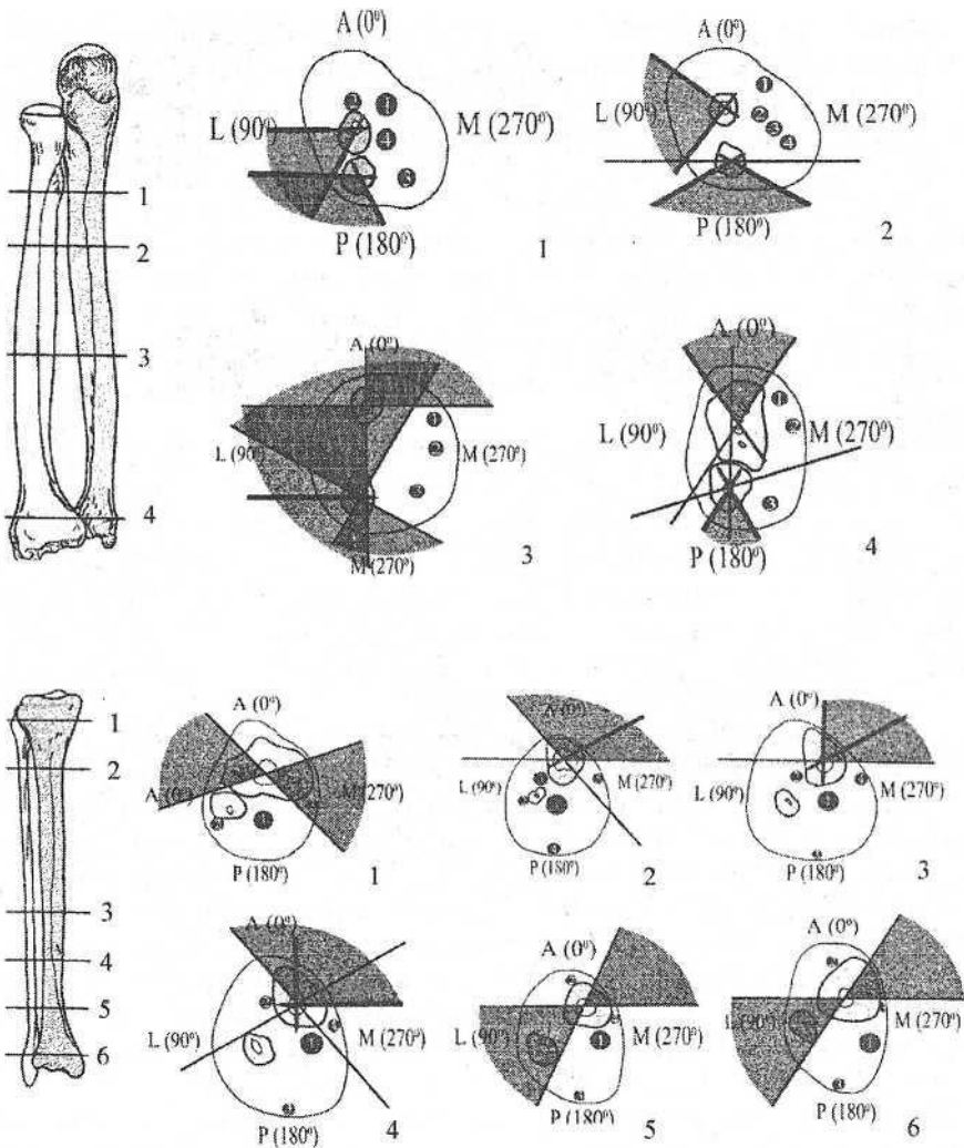
Рис. 44. Секторы безопасного проведения спиц на различных уровнях предплечья ( 0^\circ — фронтальная плоскость, лучевая сторона) и голени ( 0^\circ — сагиттальная плоскость, передняя сторона)
