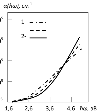
1-rasm 1-(18), 2-(19) va 3-(20) formulalardan hisoblangan zonalararo yutilish spektrlari.
