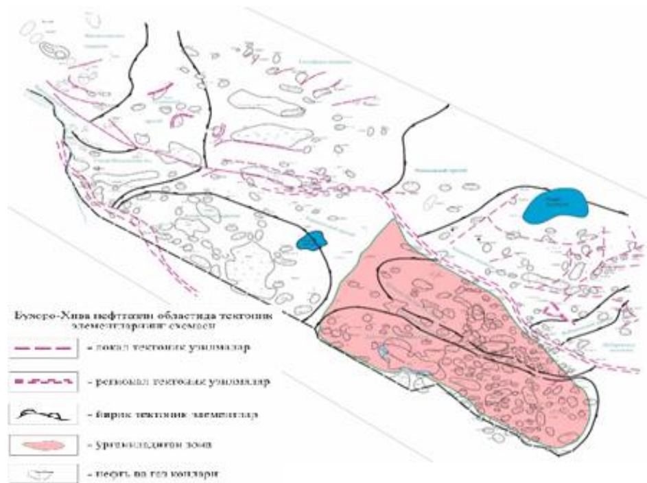
1-rasm. Buxoro-Xiva neftgazli oblastida tektonik elementlarning sxemasi
